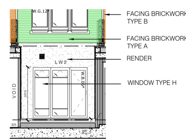
Elevation 2A Scale 1:100
