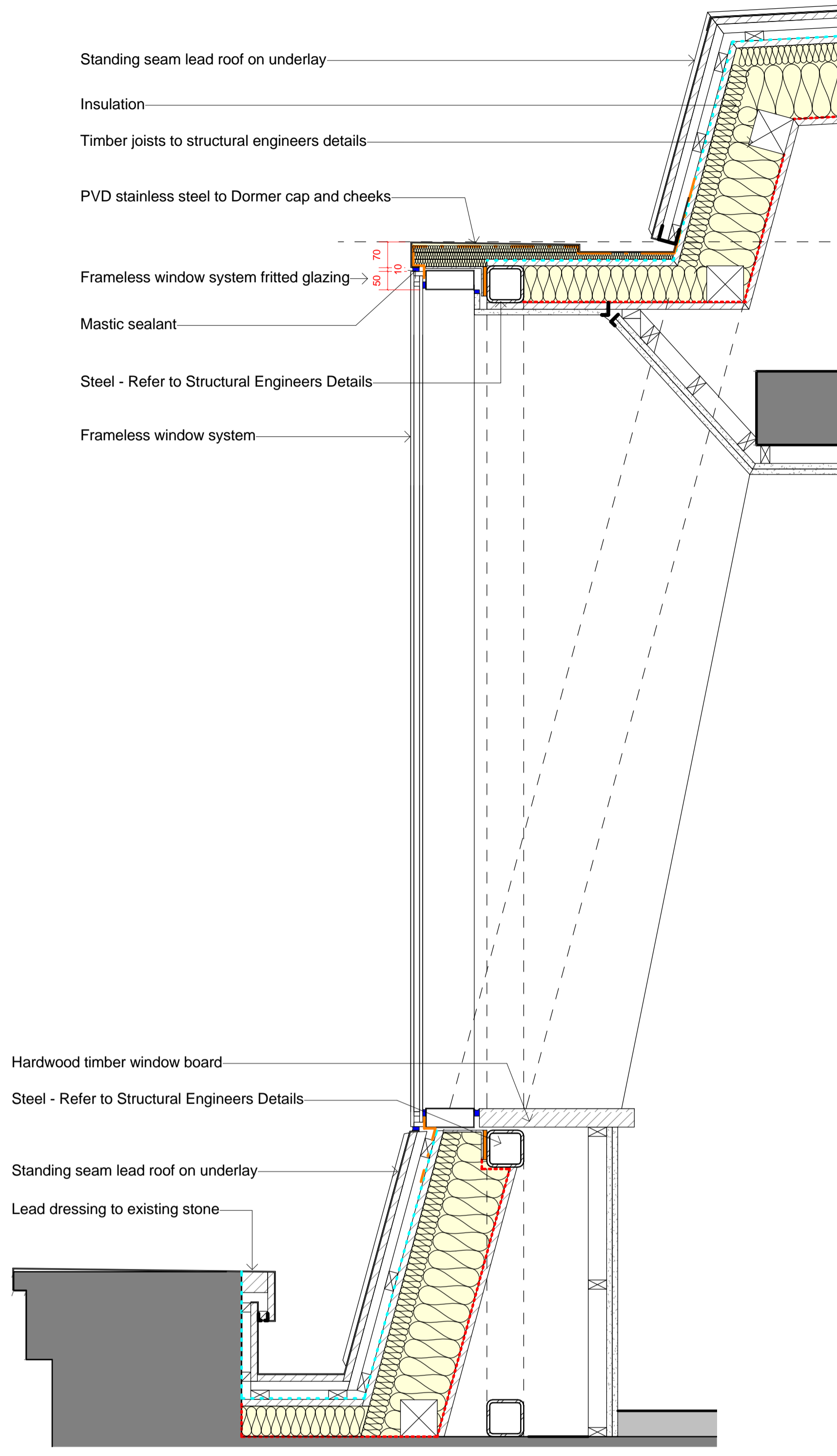
1 25 DMS Dormer Section Detail Scale: 1 : 10
