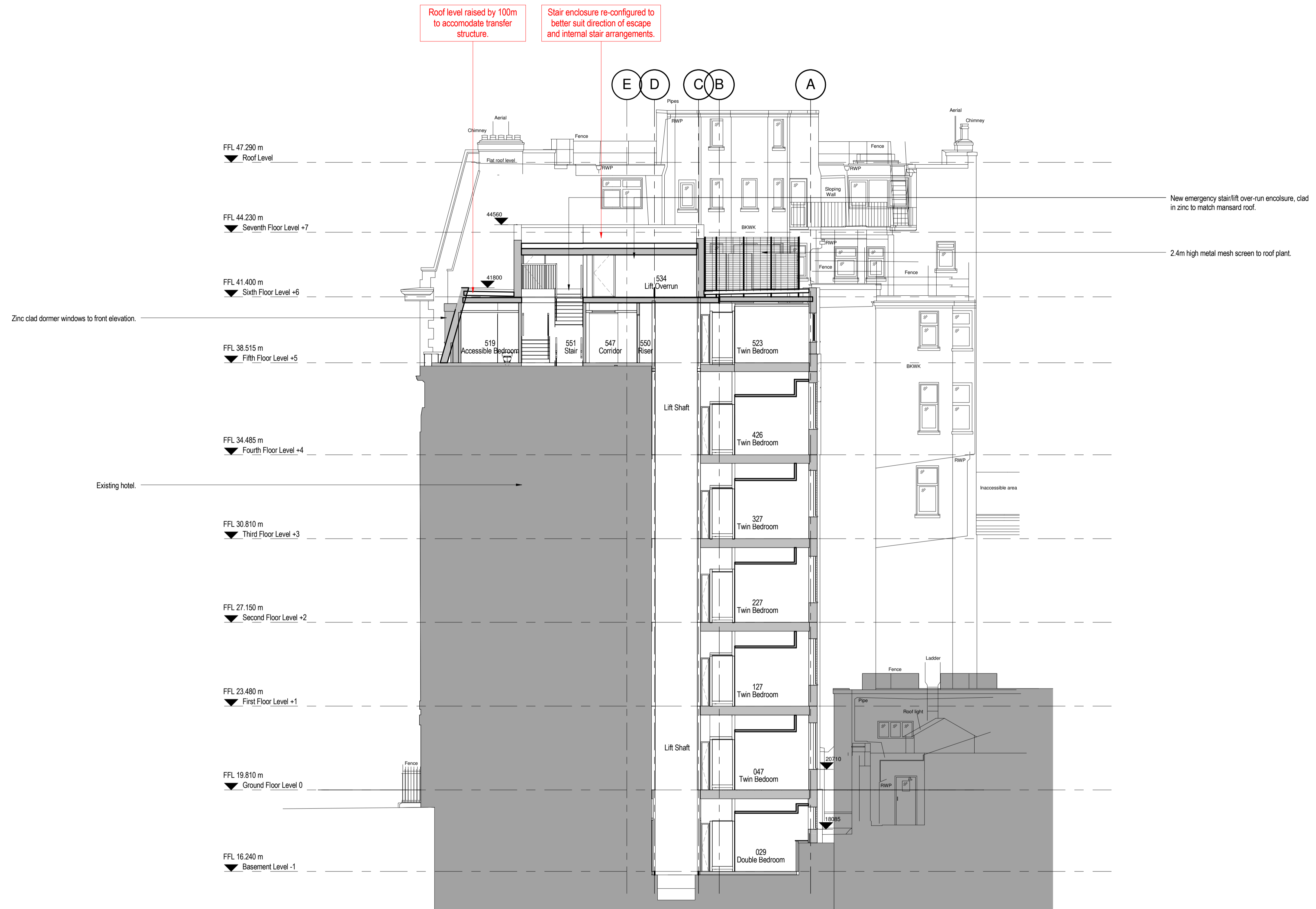
GA Section B-B 1 : 100
