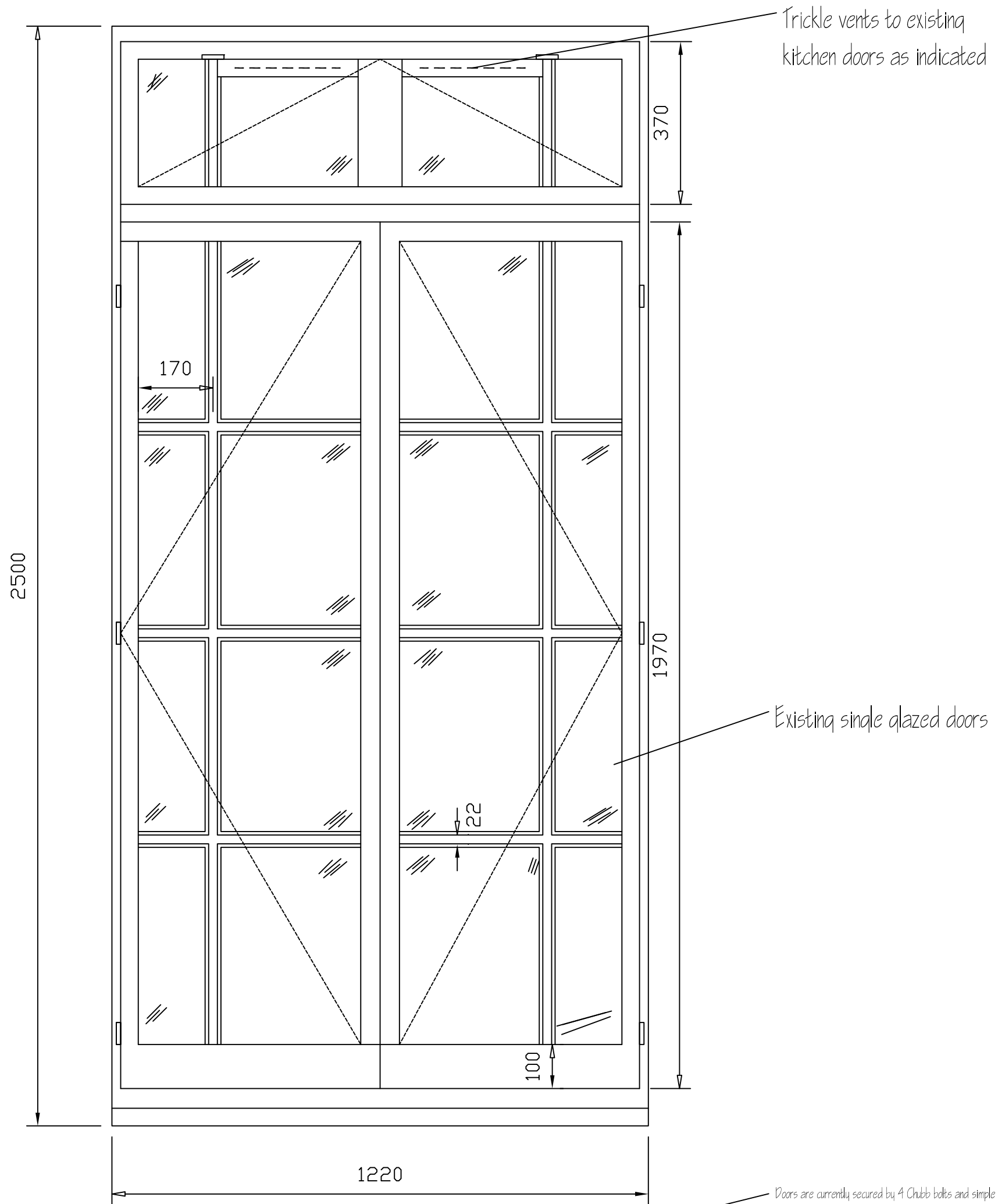
ELEVATION
