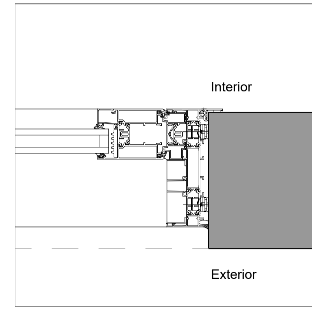
JAMB (DOOR)
