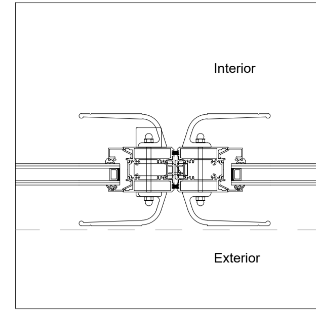
DOOR MEETING EDGE
