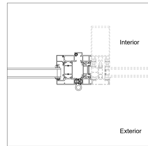
JAMB
