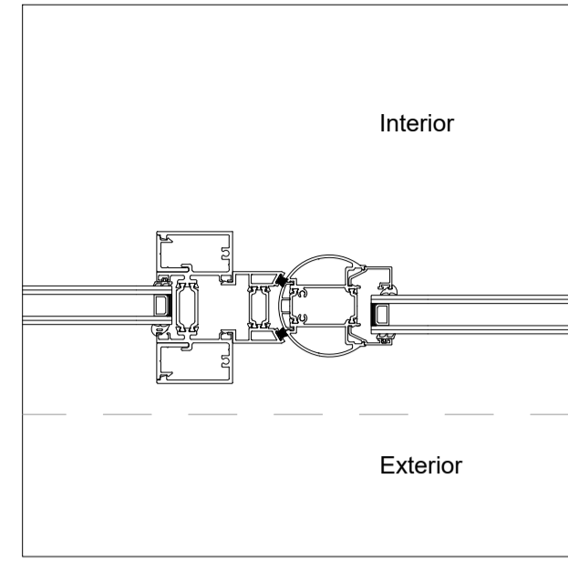
MULLION/DOOR JAMB
