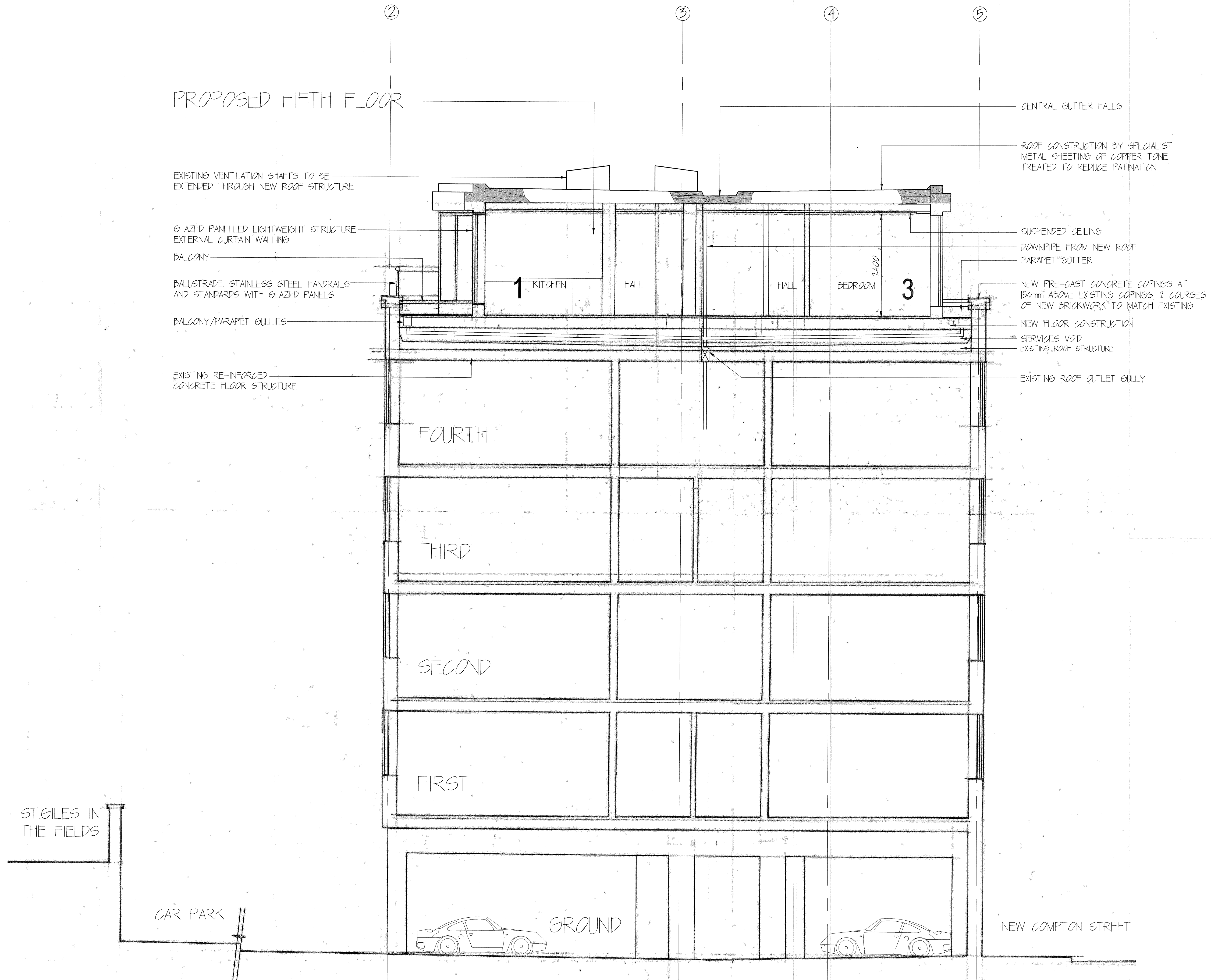
SECTION X-X (N.T.S.)
