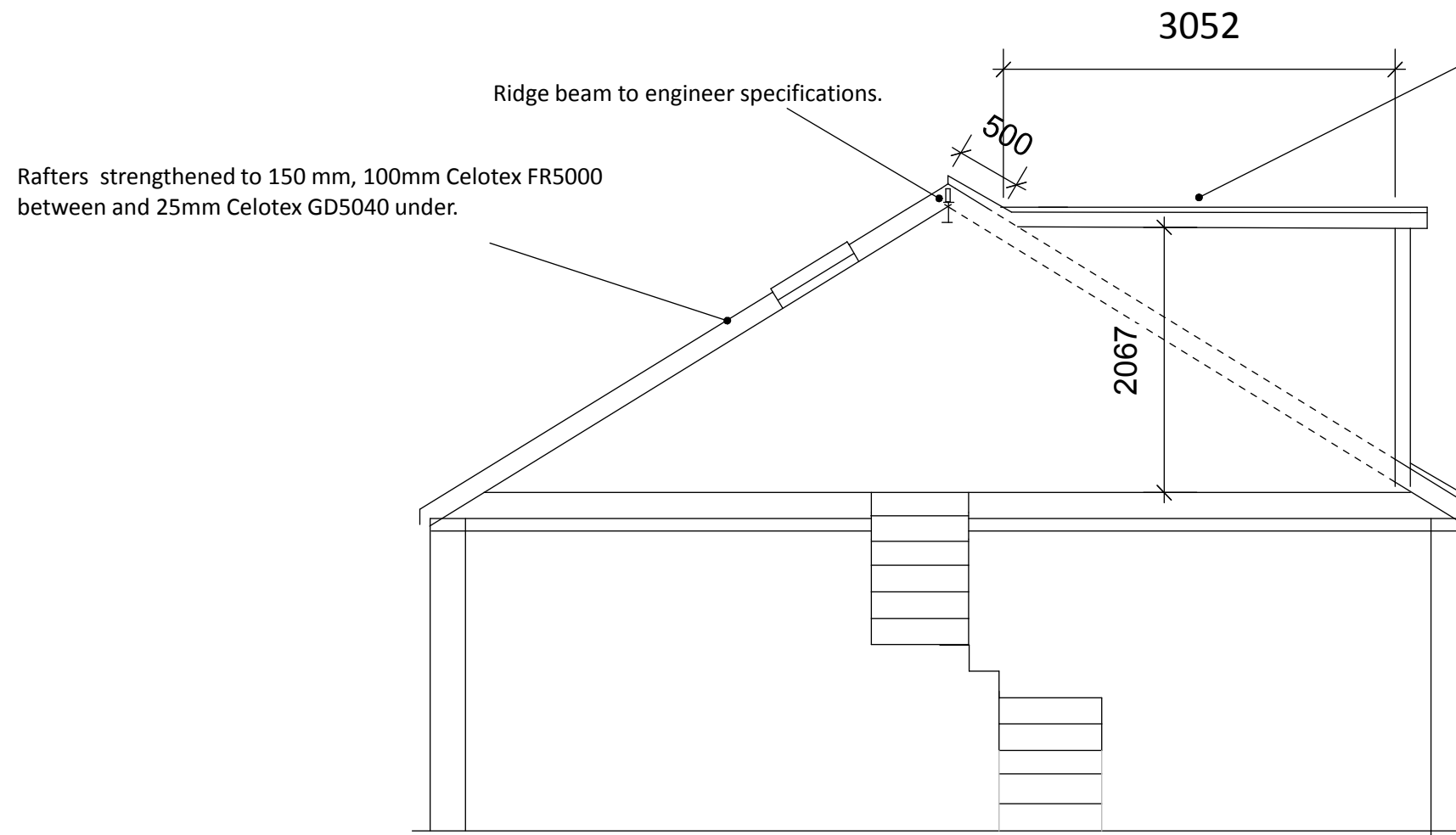
Section Scale: 1:50
