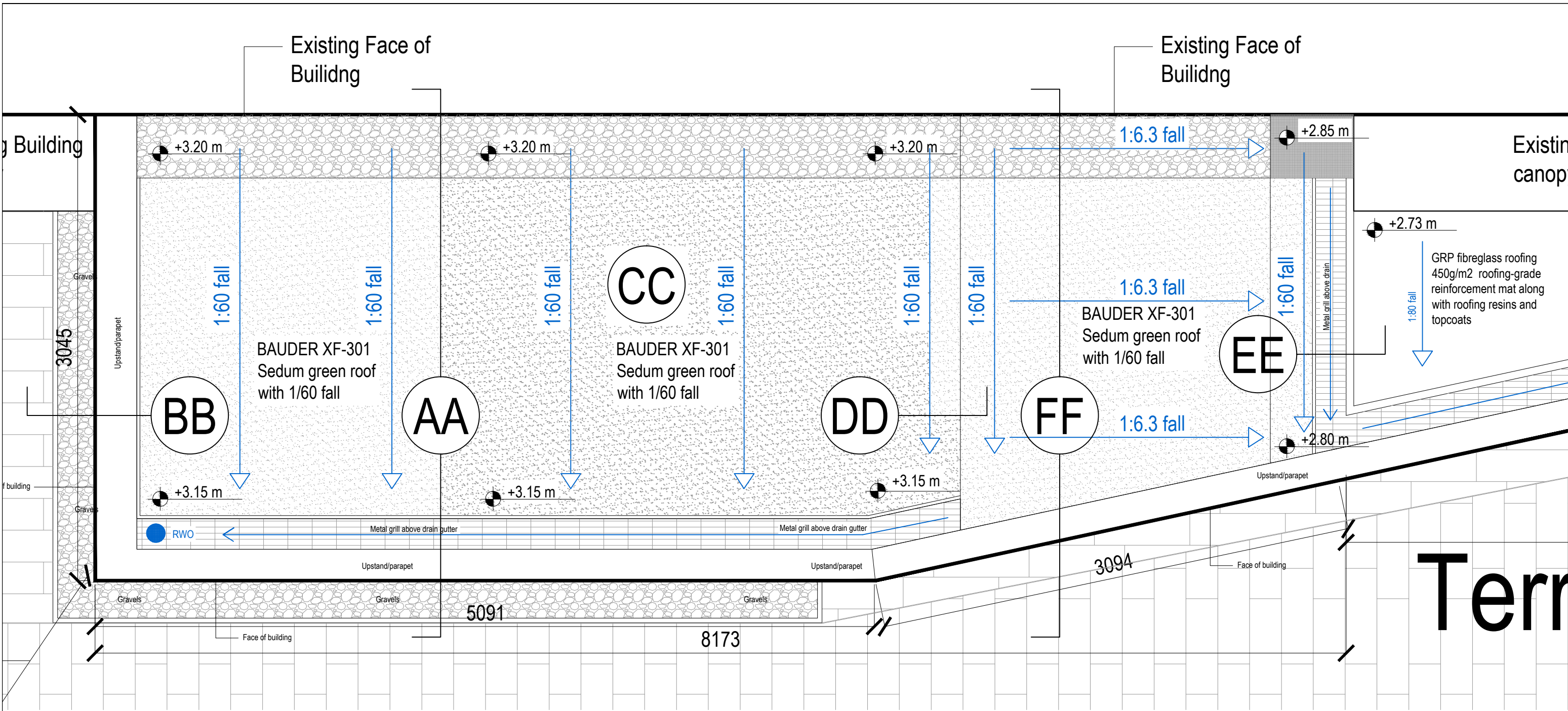
1 Roof Plan 1/25
