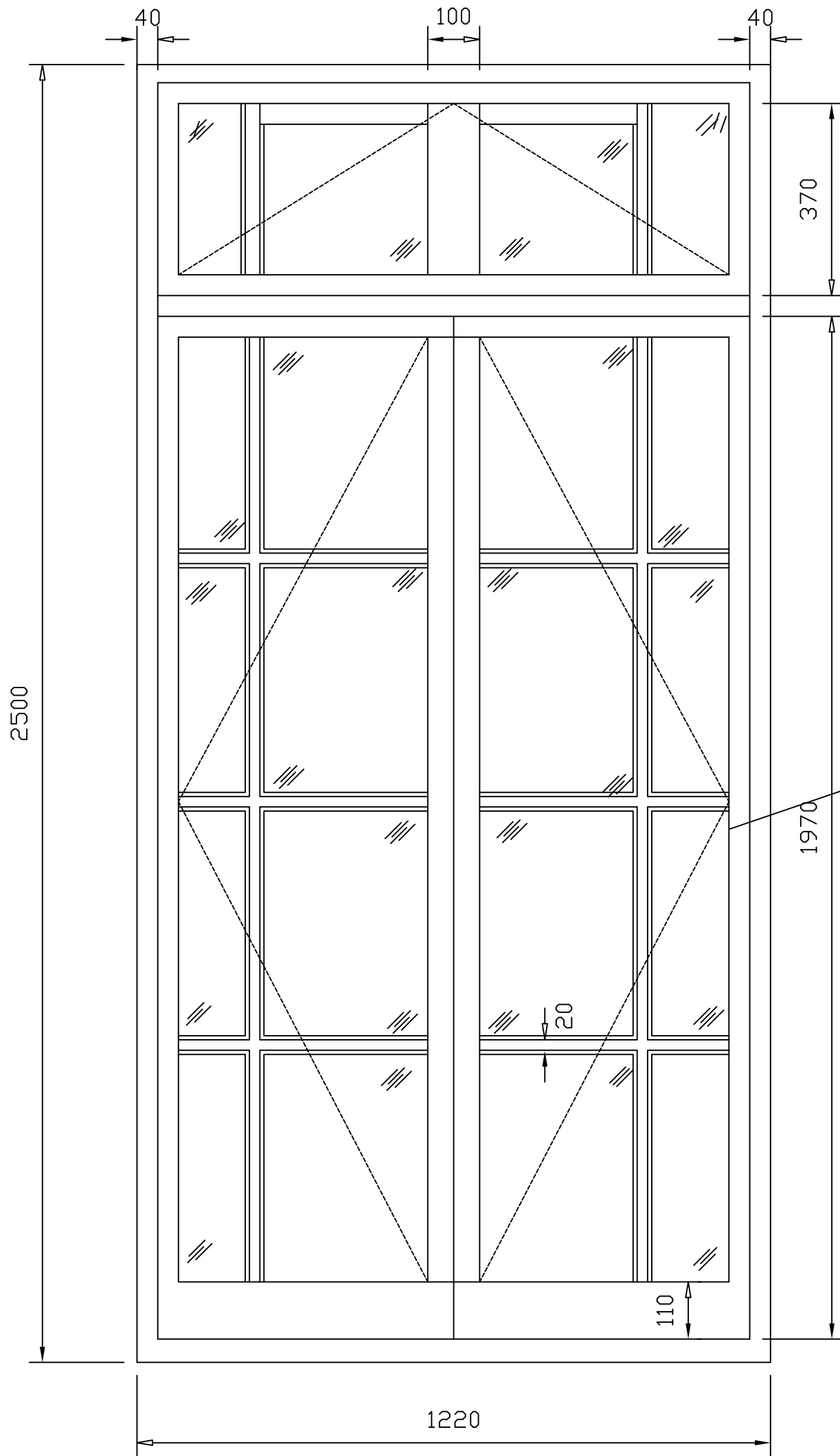
ELEVATION
