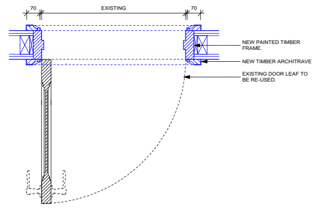
02 INTERNAL DOOR SCALE 1:10 PLAN PL-58
