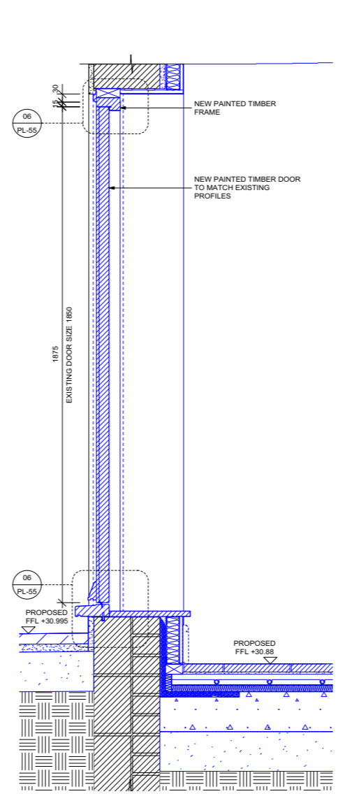
03 DOOR DL18 SCALE 1:10 SECTION PL-55
