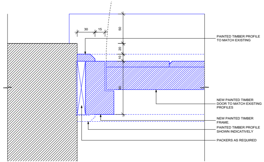
05 DOOR DL18 SCALE 1:2 JAMB DETAIL PL-55
