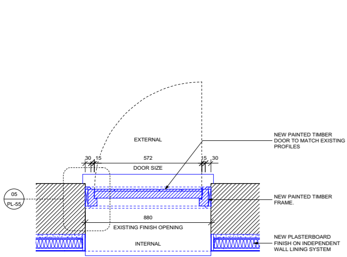
04 DOOR DL18 SCALE 1:10 PLAN PL-55
