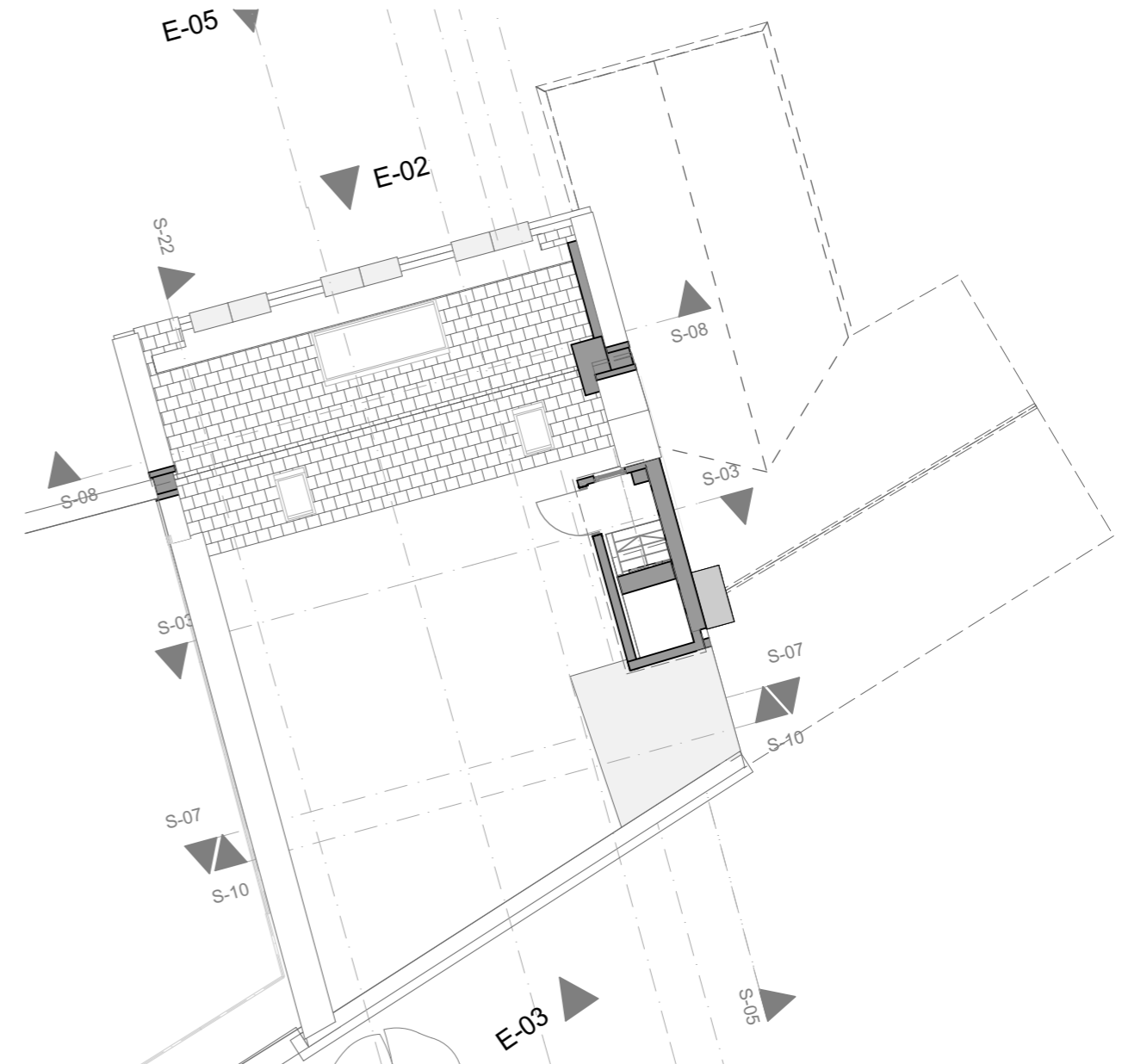
3. RF-Roof Fl 1:100
