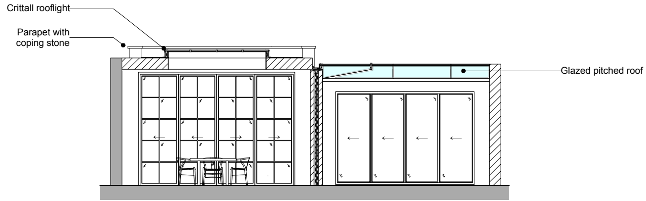
SECTION DD
