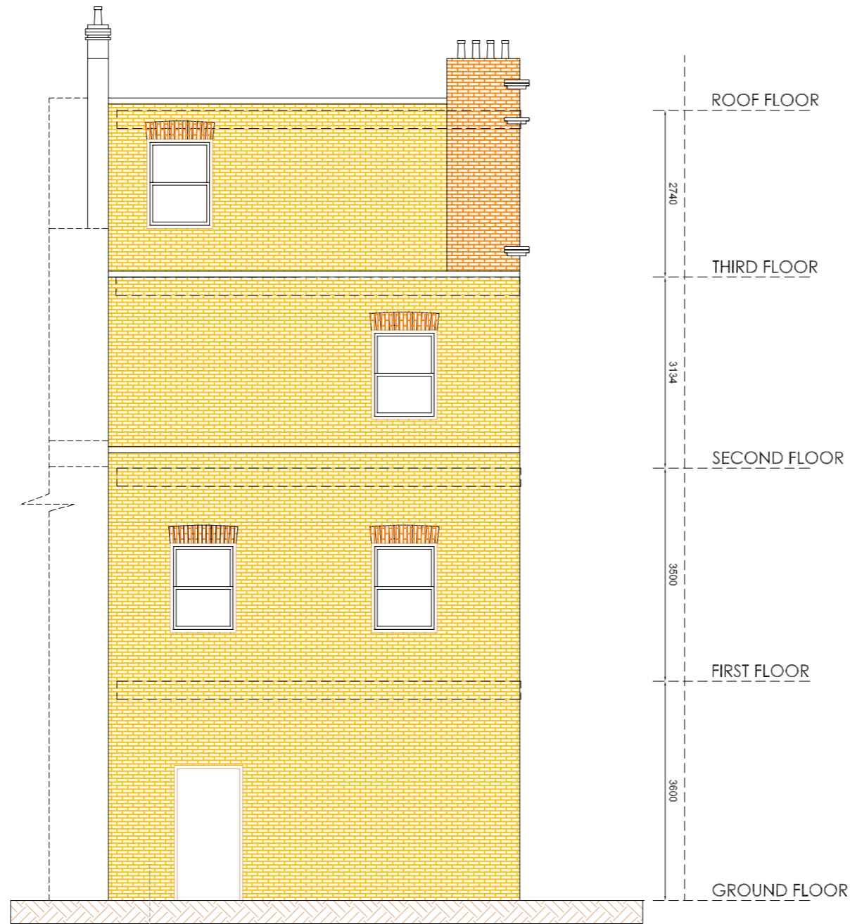
C EXISTING REAR ELEVATION Scale: 1:100
