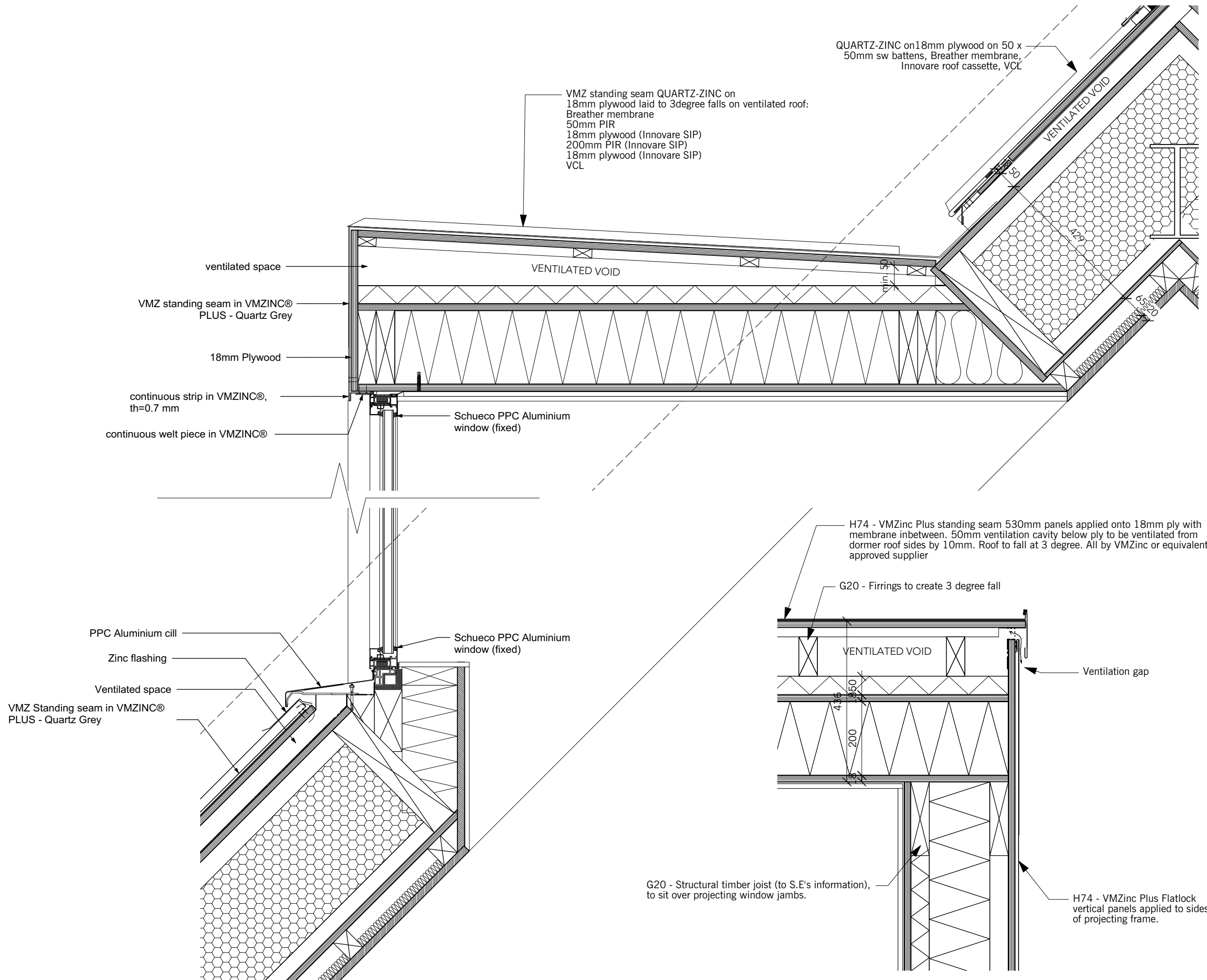
01 Dormer Section D208
