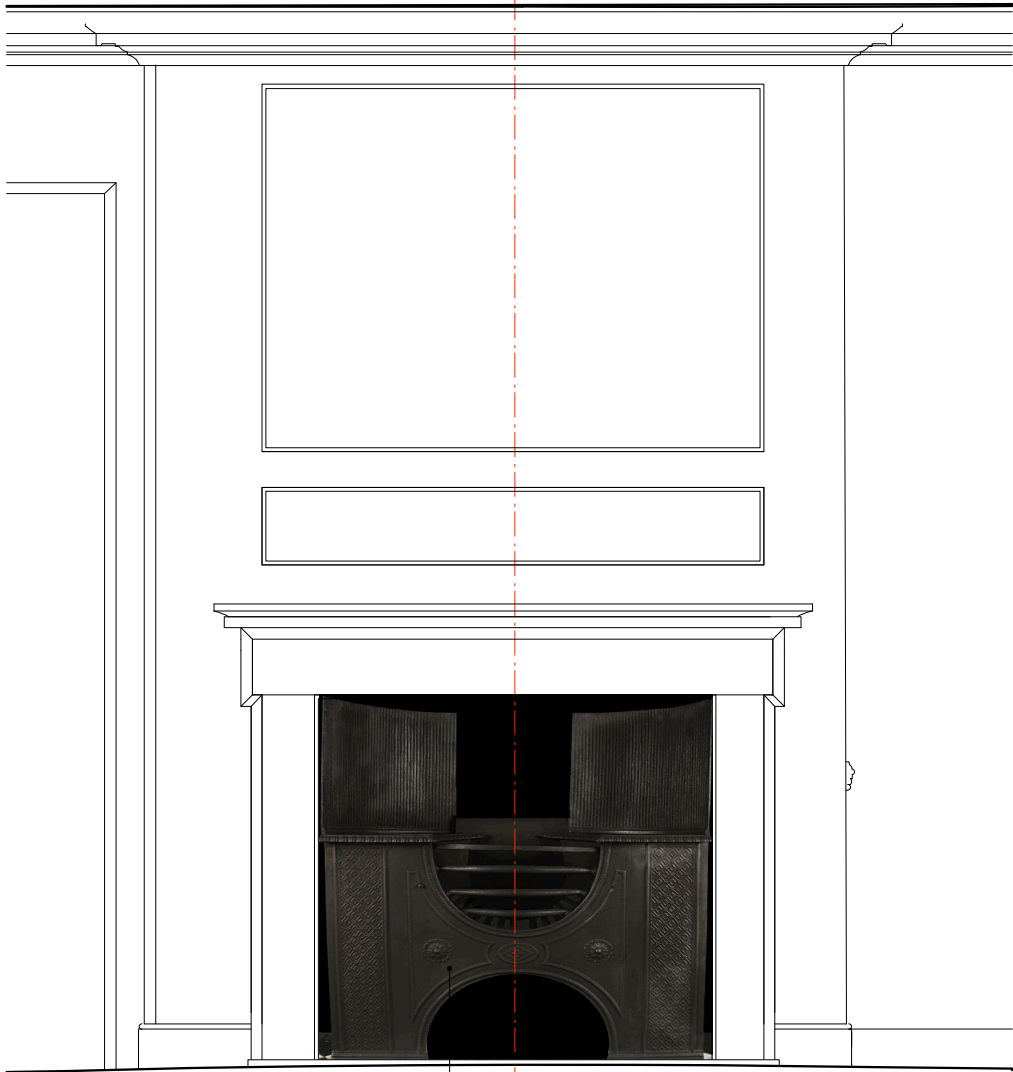
ELEVATION
