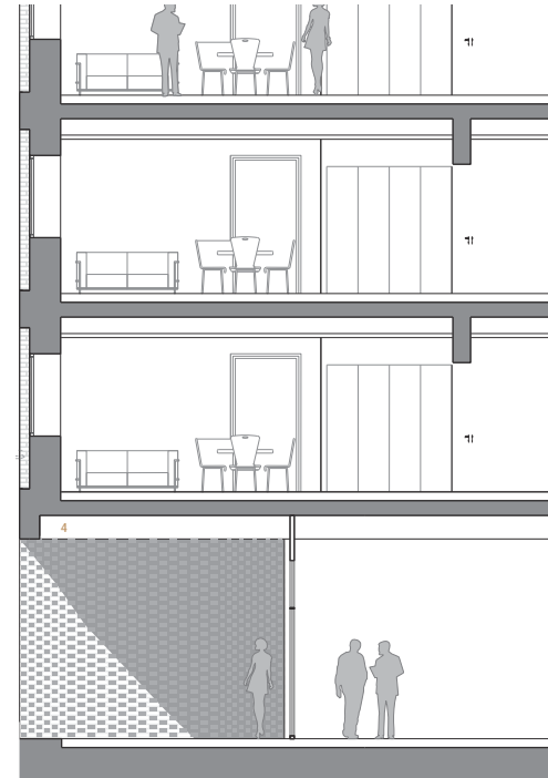
2.4 Section D-D
