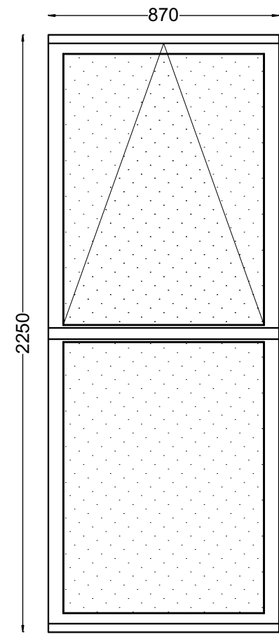
ELEVATION
