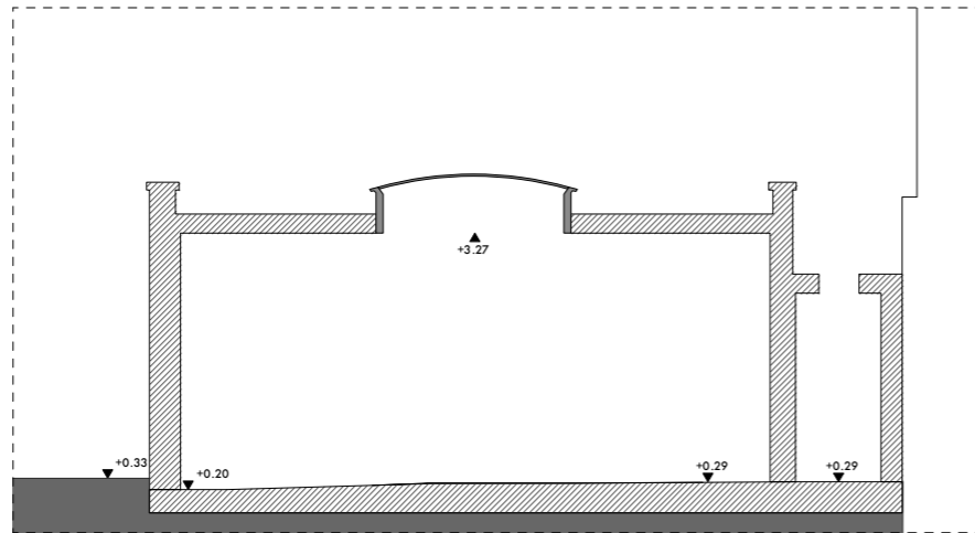
Section DD
