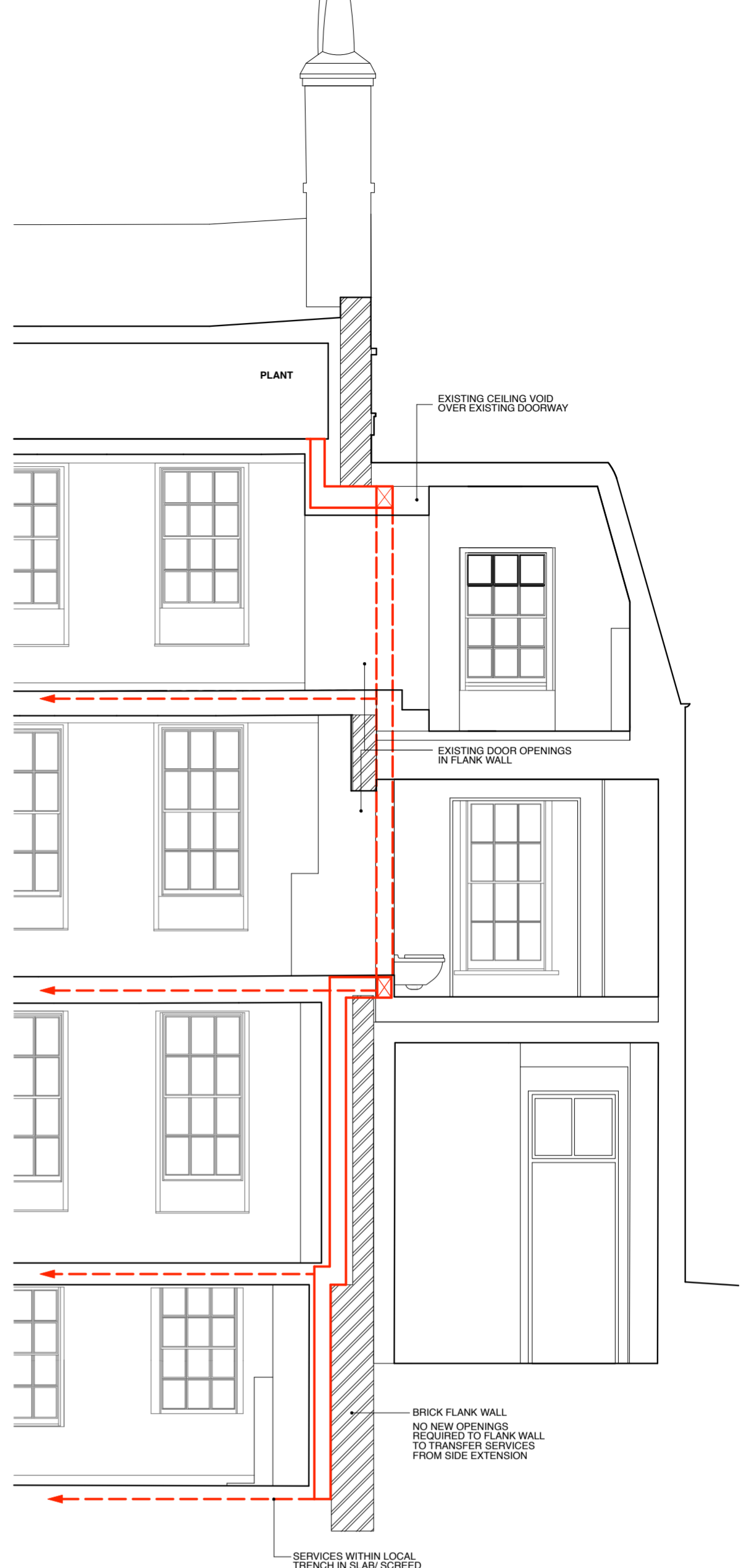
SECTION XX 1:50
