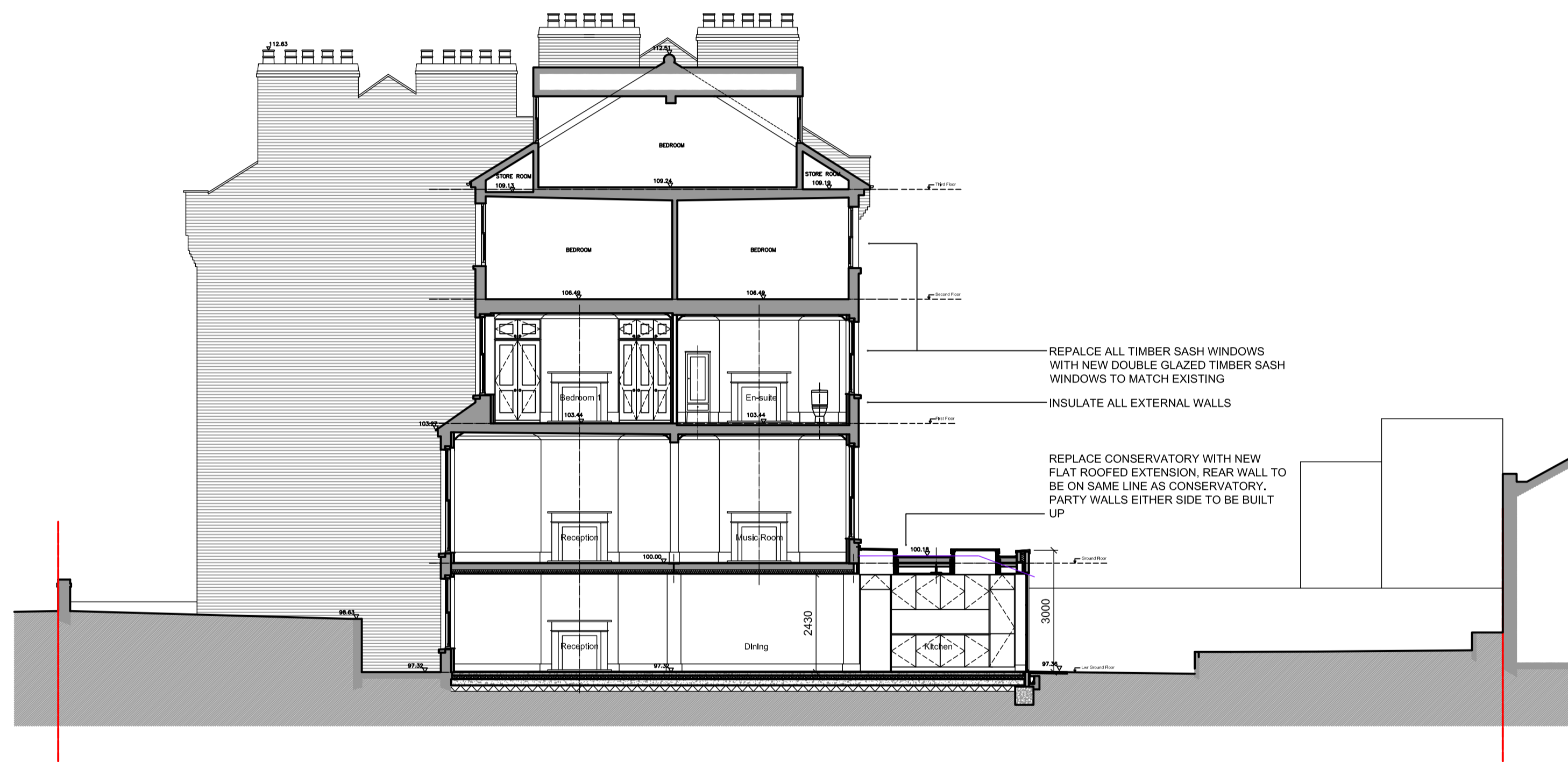
Section A-A
