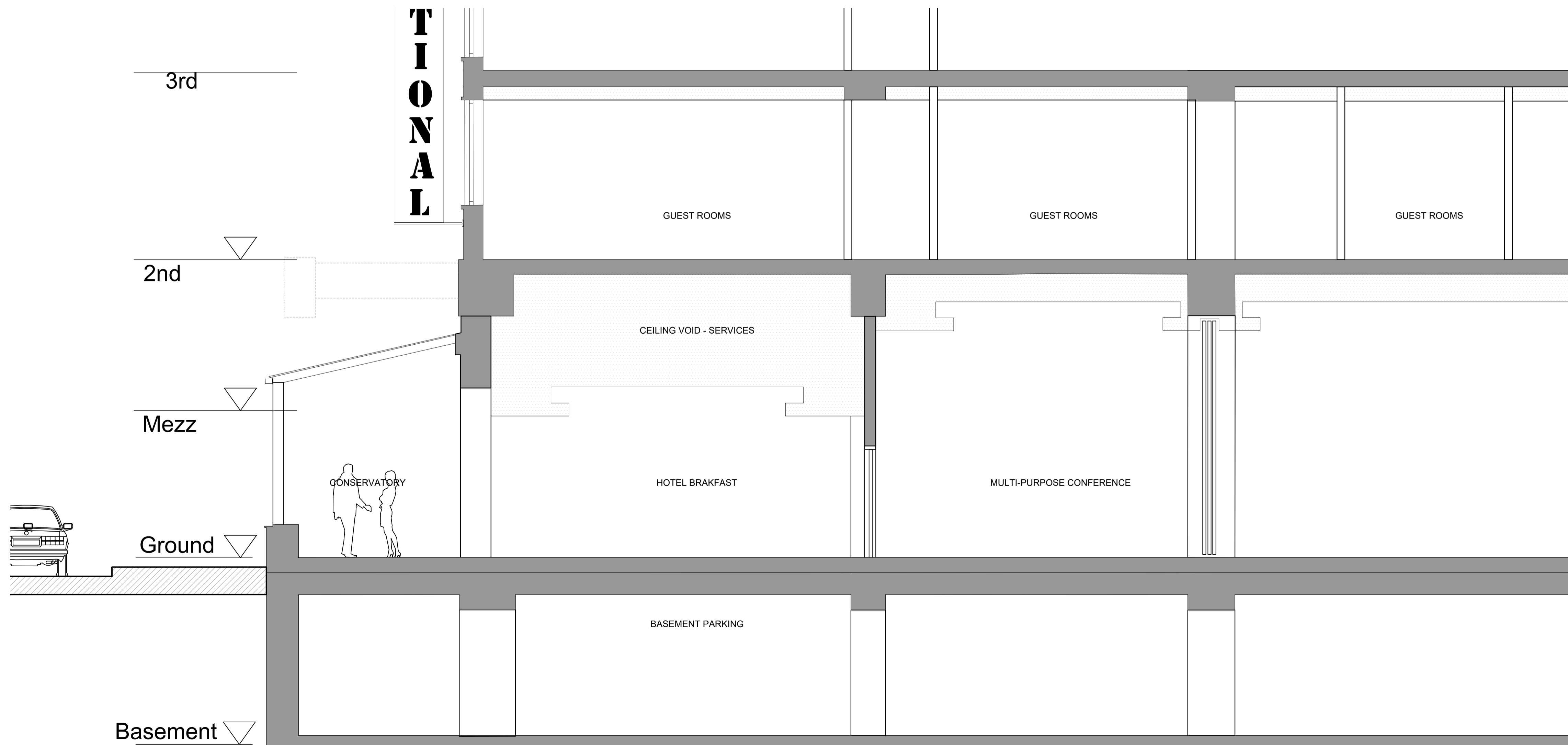
3 SECTION 3-3 Scale: 1:50 @ A1
