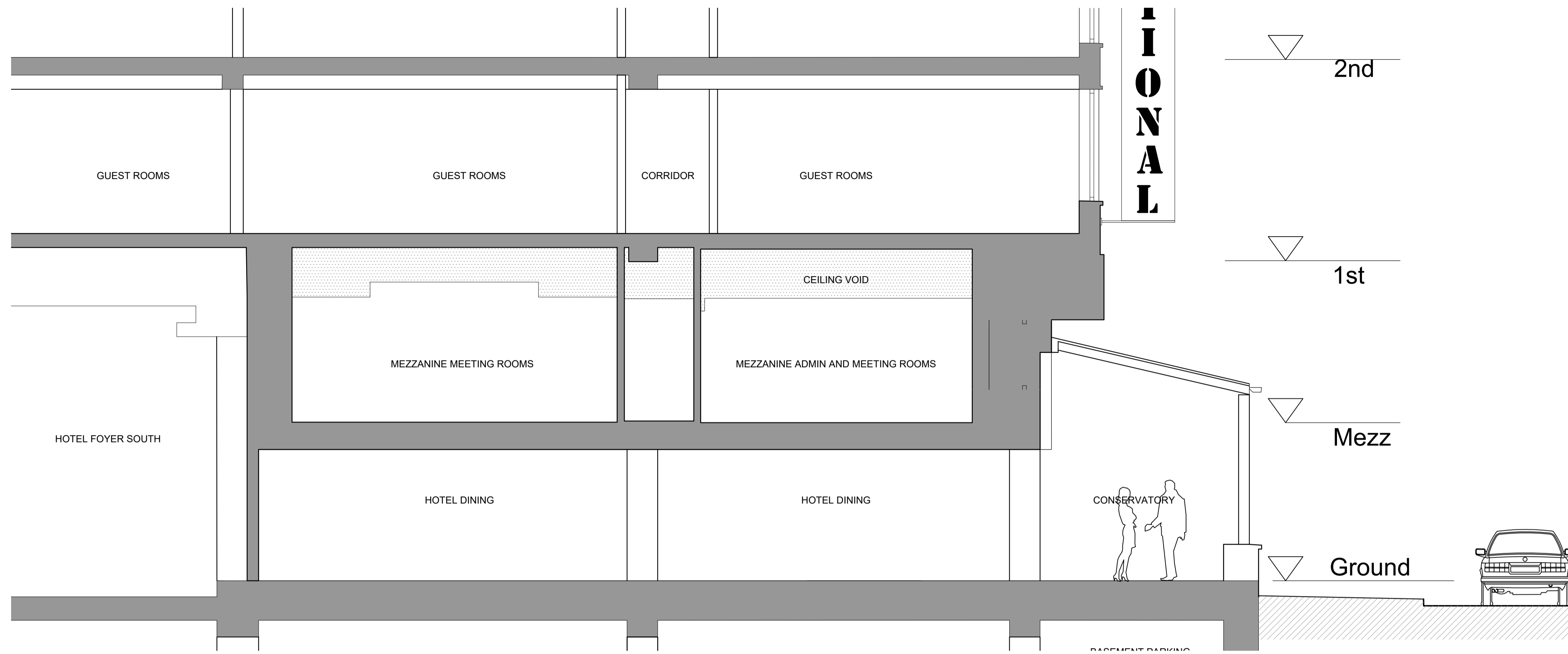
4 SECTION 4-4 Scale: 1:50 @ A1
