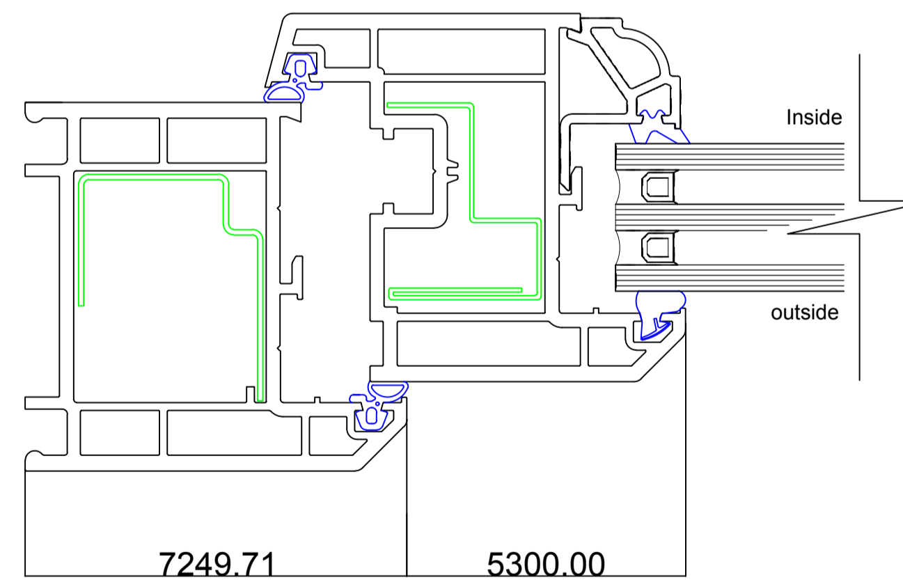
SECTION R 1:1
