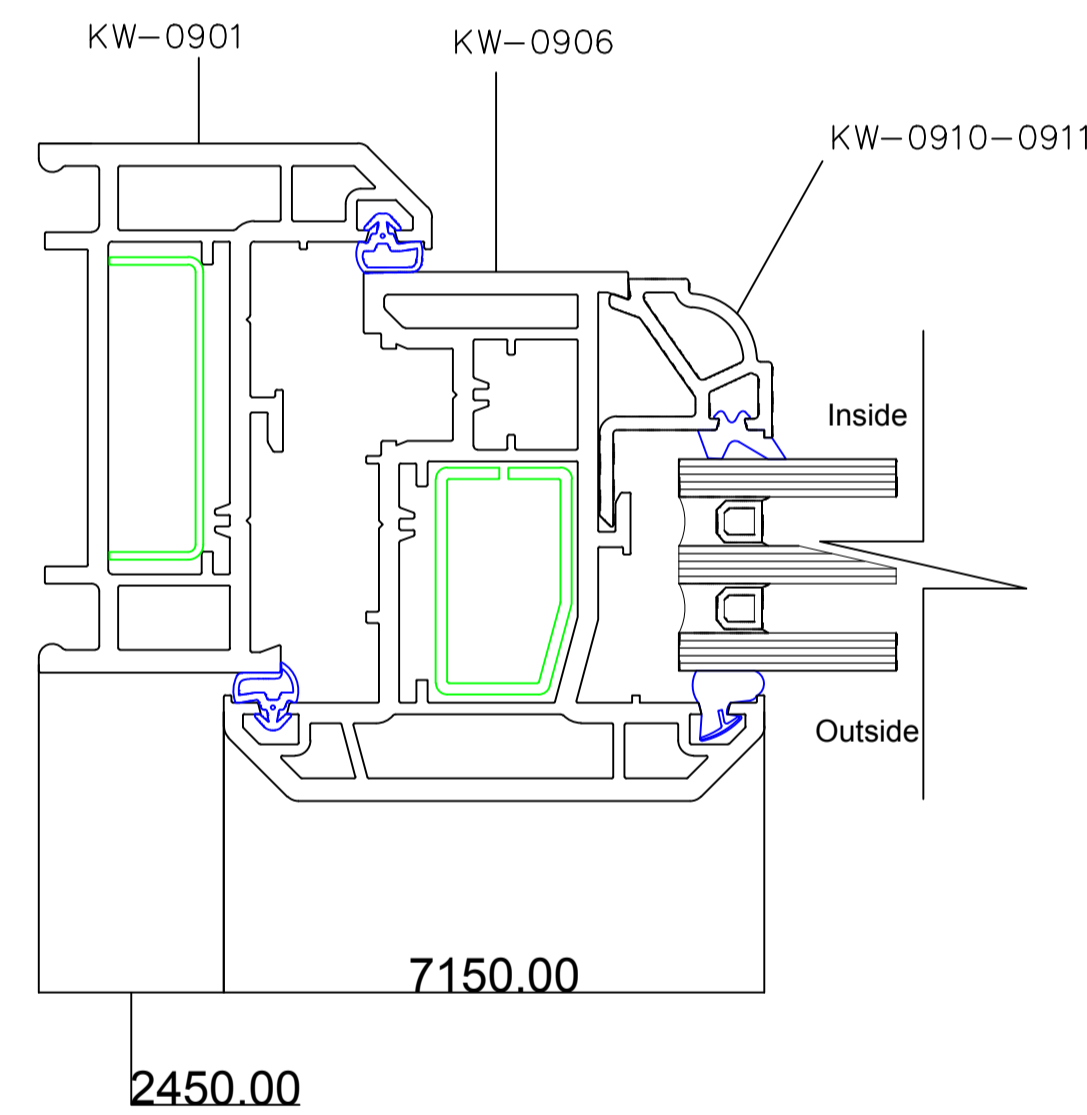
SECTION D 1:1
