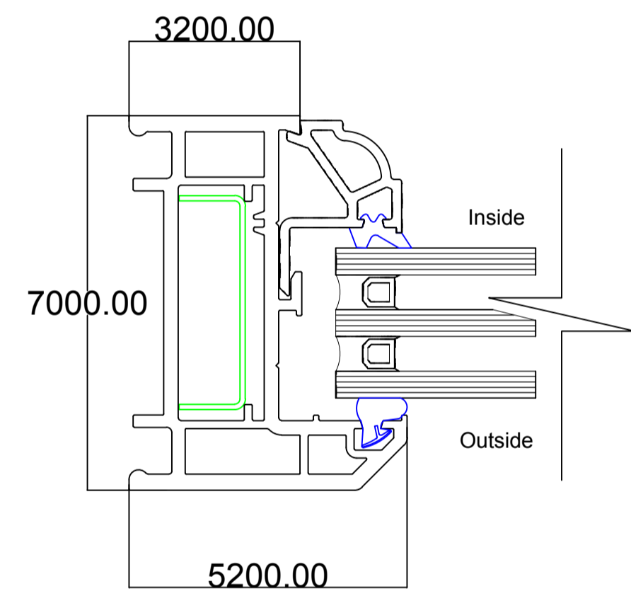
SECTION A 1:1
