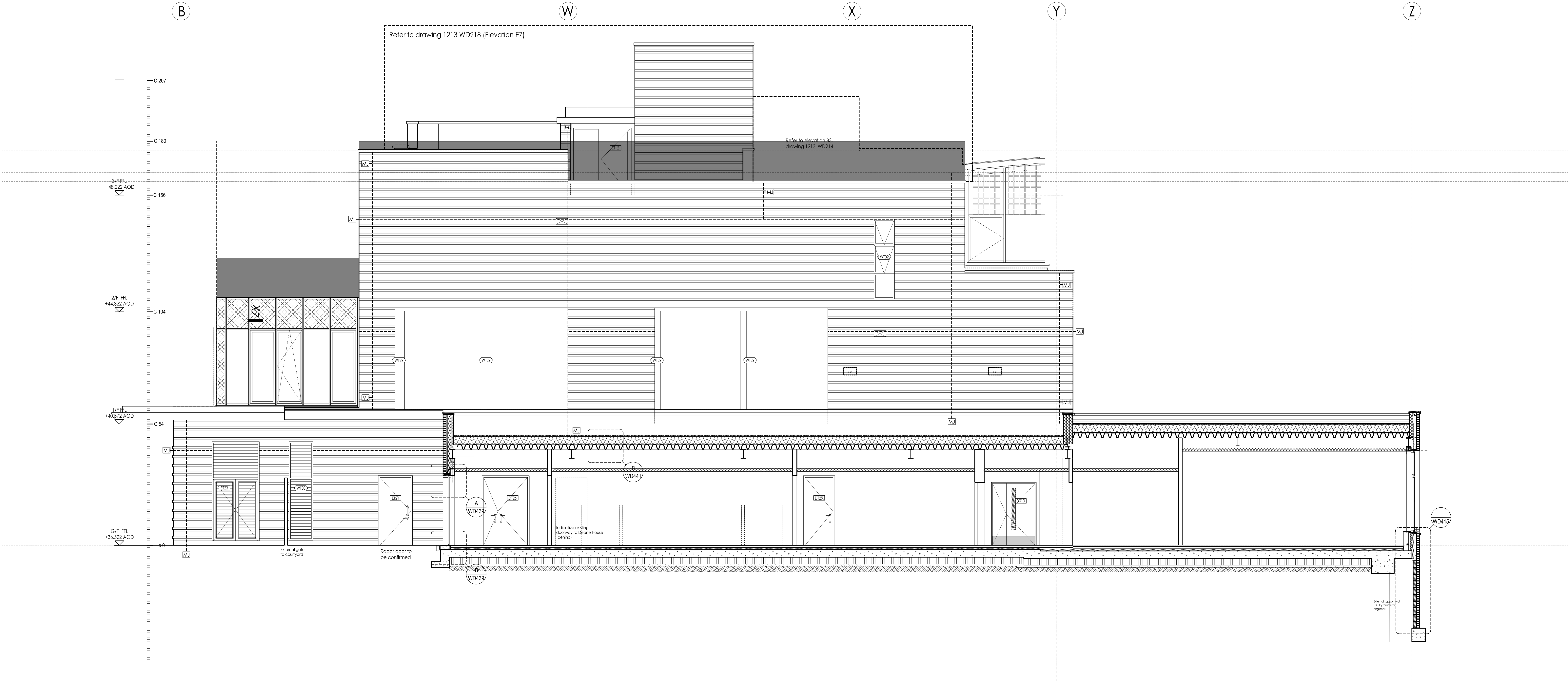
D1 Elevation
