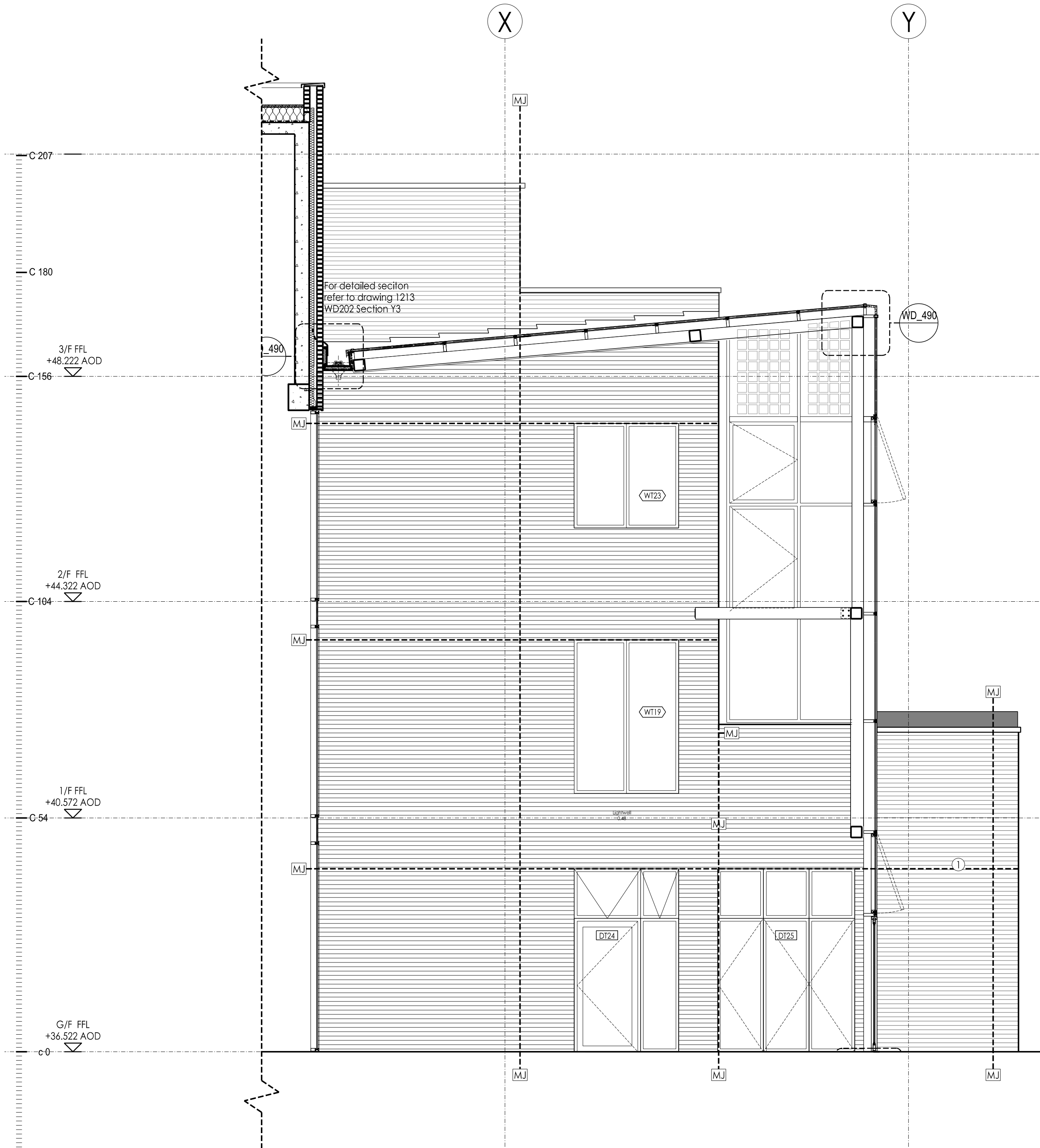
B3 Elevation
