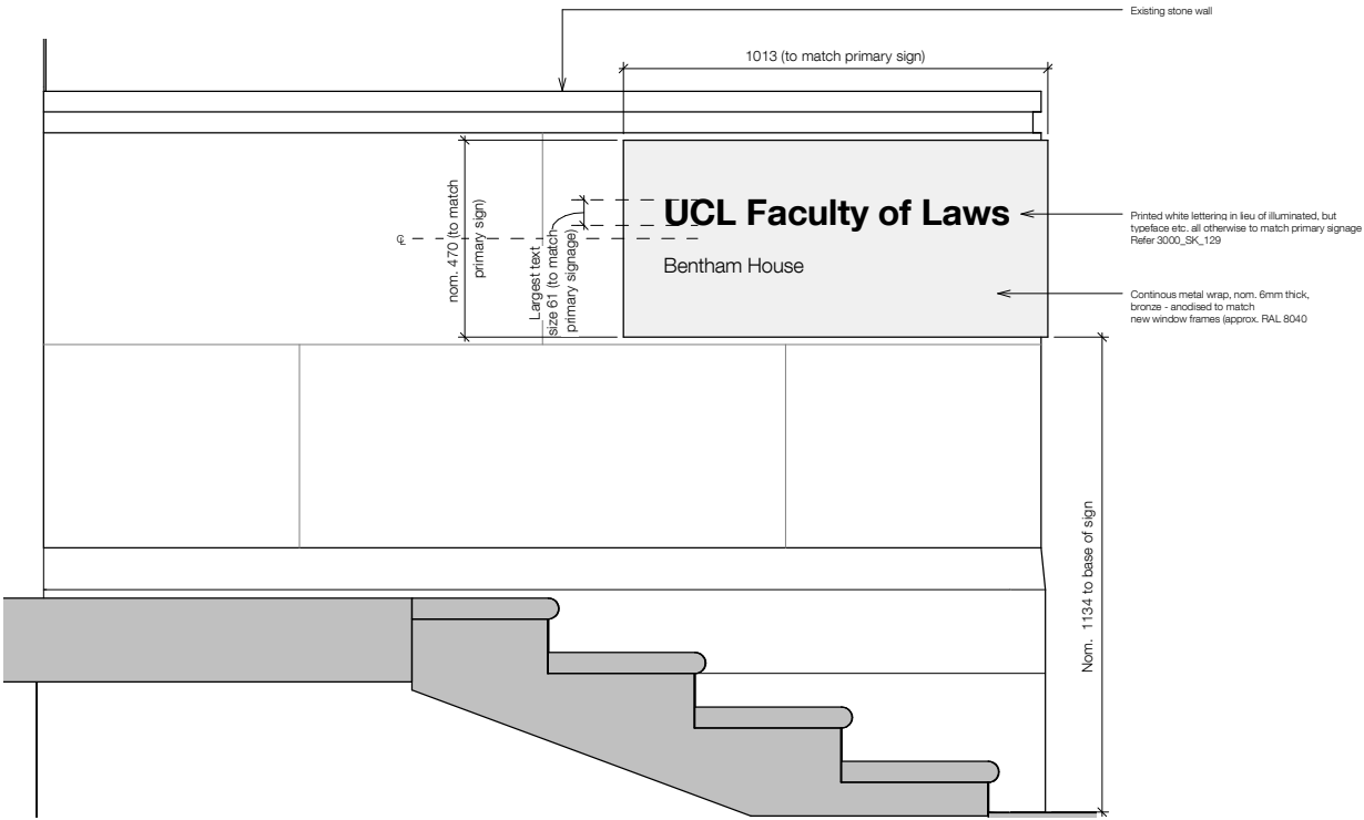
1 New Signage Elevation 1 1 : 10
