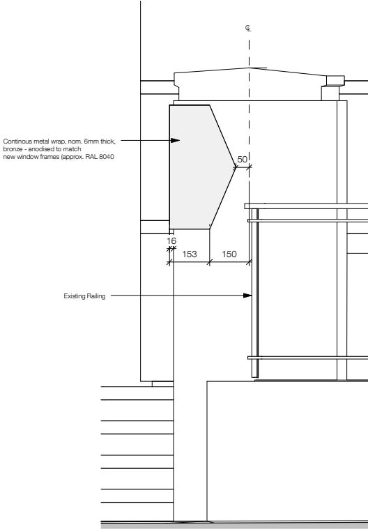
2 New Signage Elevation 2 1 : 10
