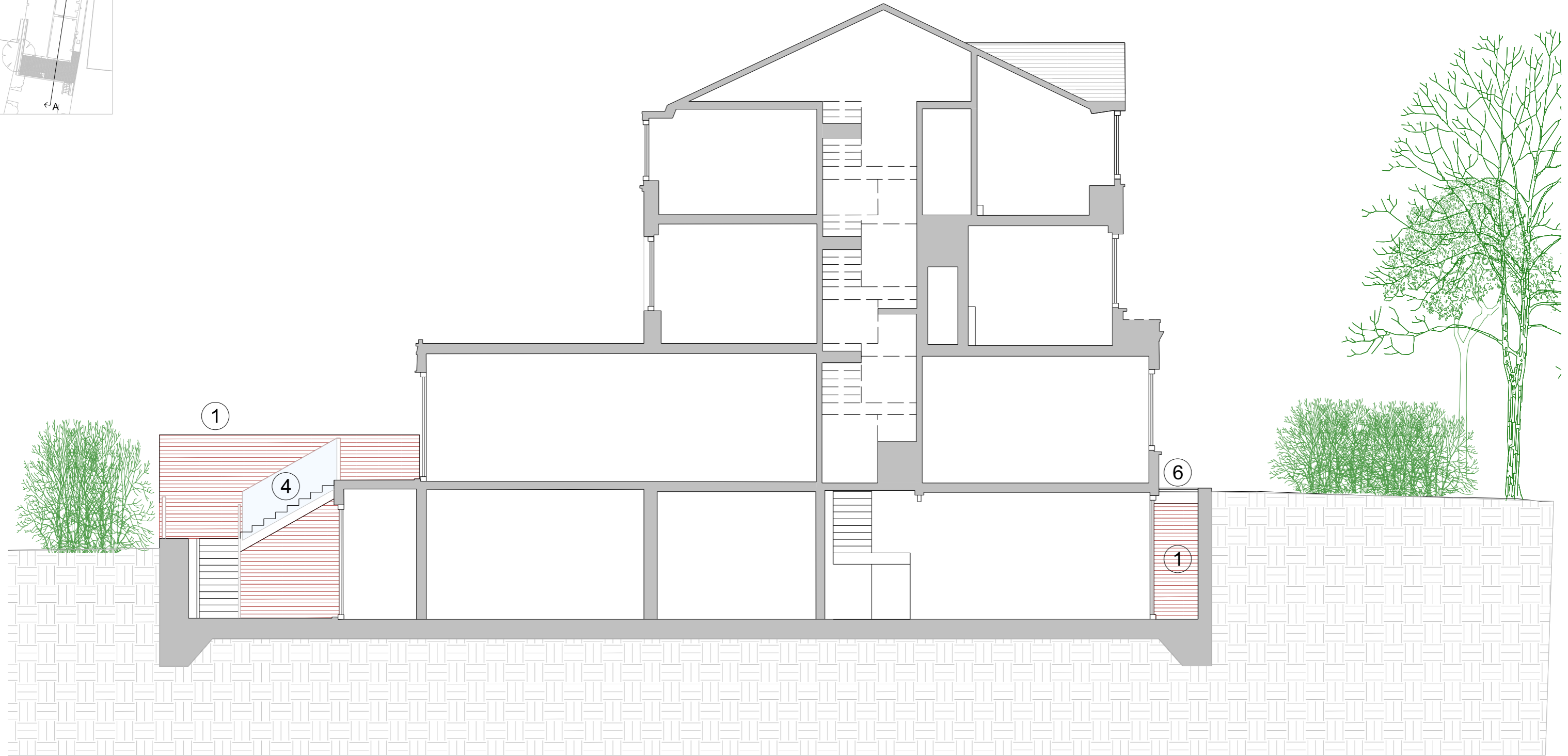
Section A-A
