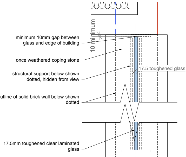
2 Plan detail Scale: 1:10
