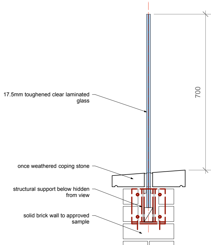
3 Section detail Scale: 1:10
