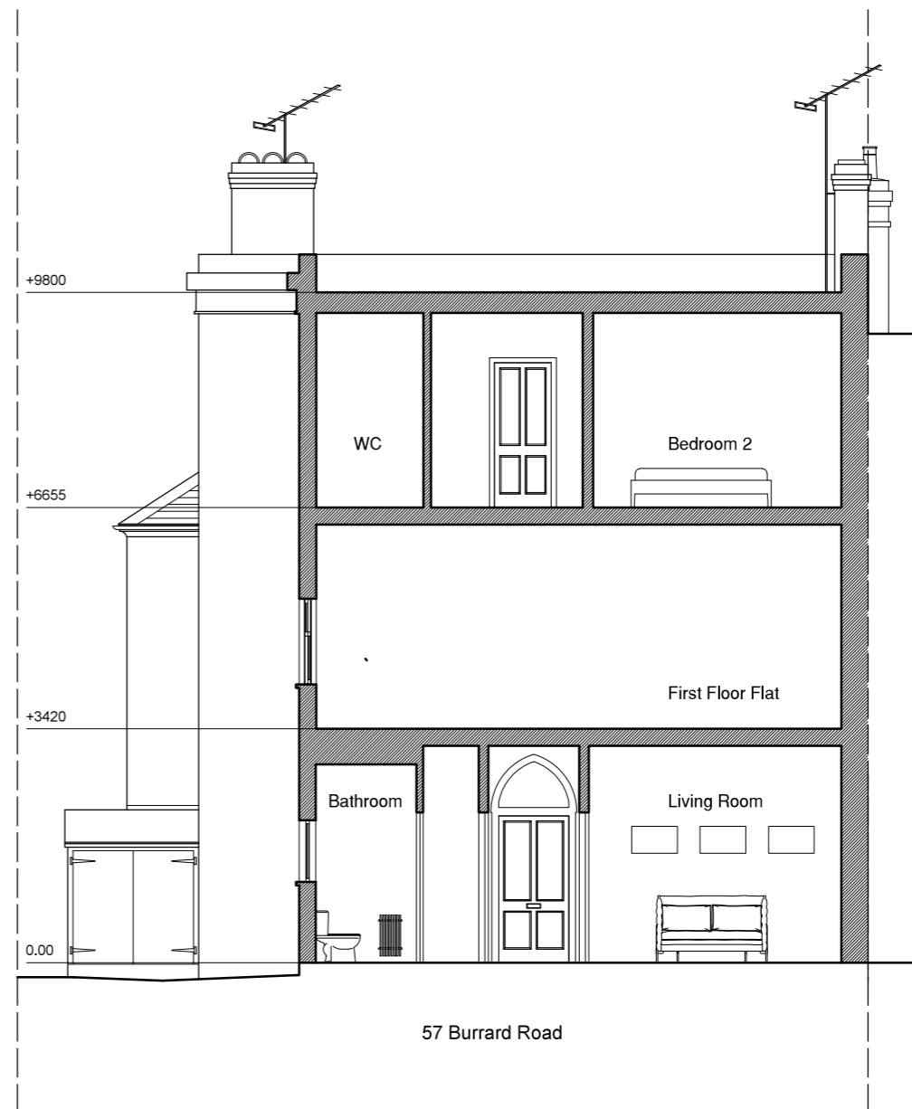
SECTION A-A
