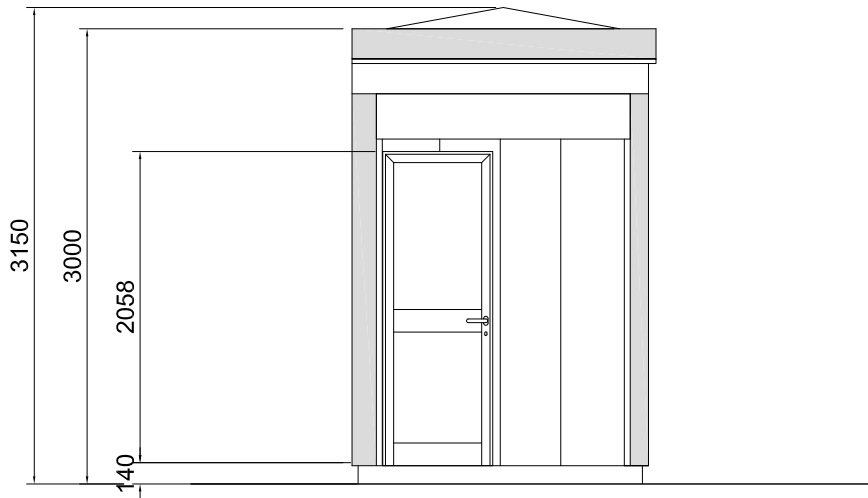
Elevation B
