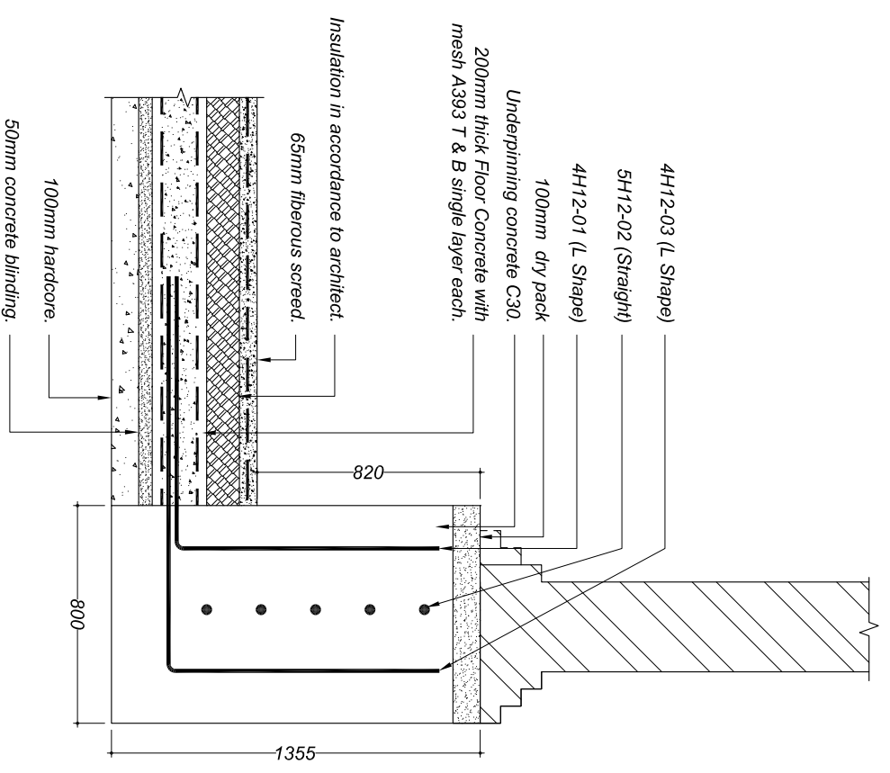
SEC S1 - S1 1:25
