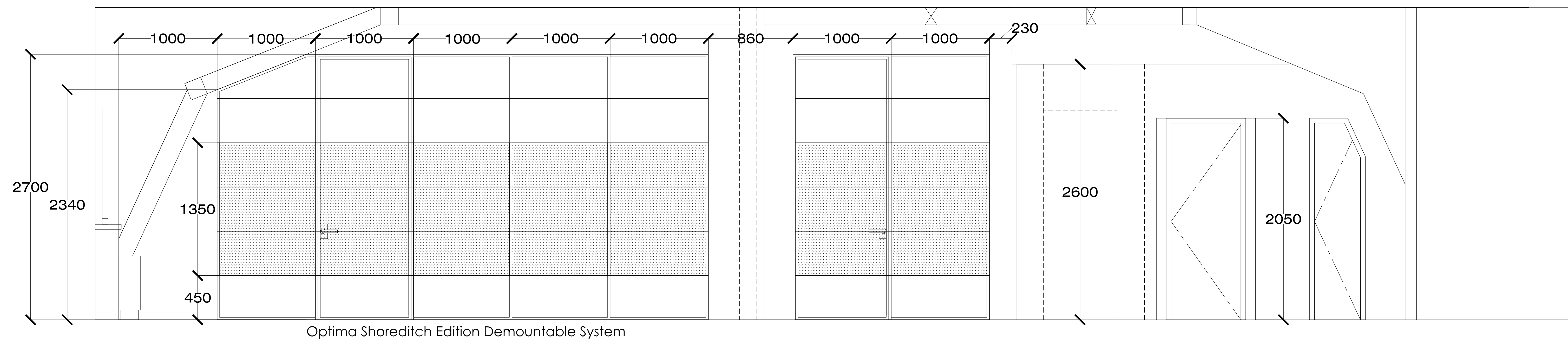
ELEVATION BB
