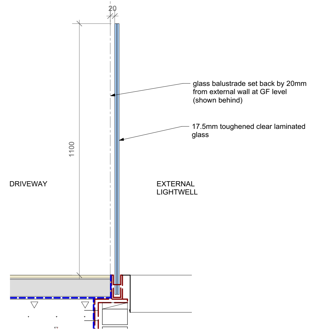
2 balustrade_section Scale: 1:10
