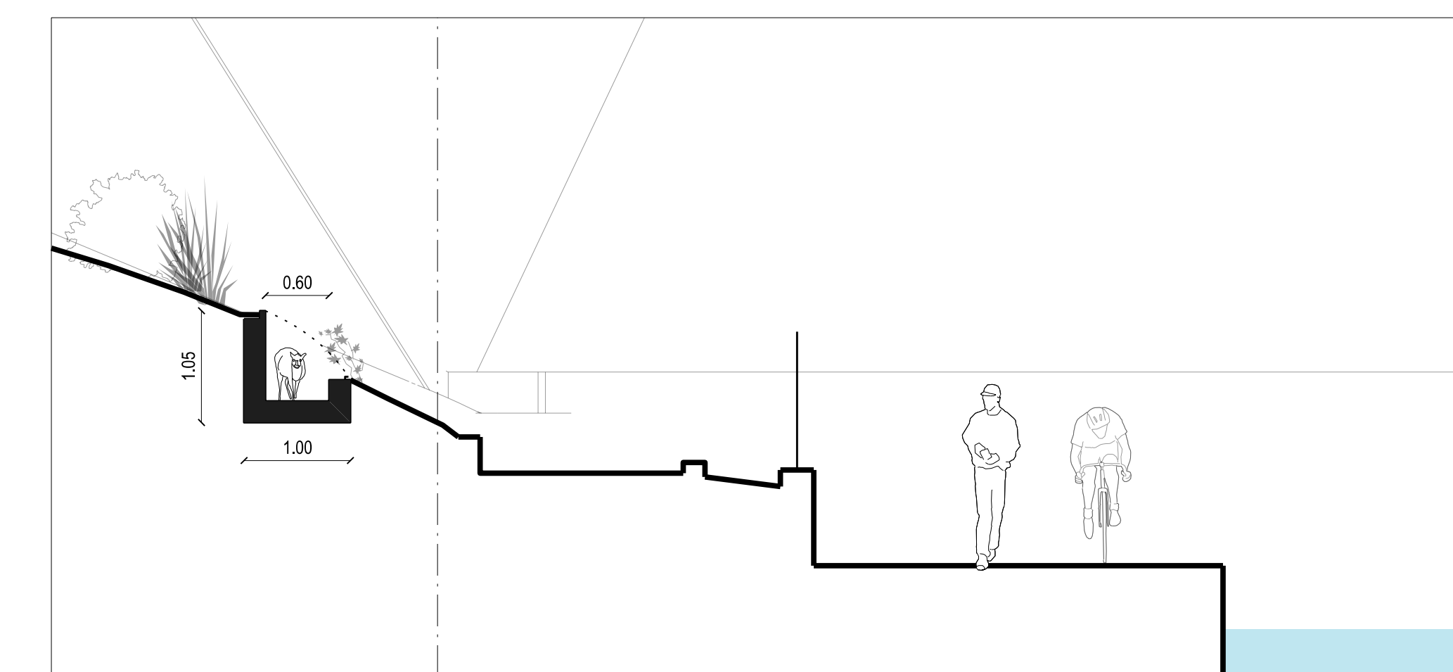
01 Section Duiker Tunnel 1:50
