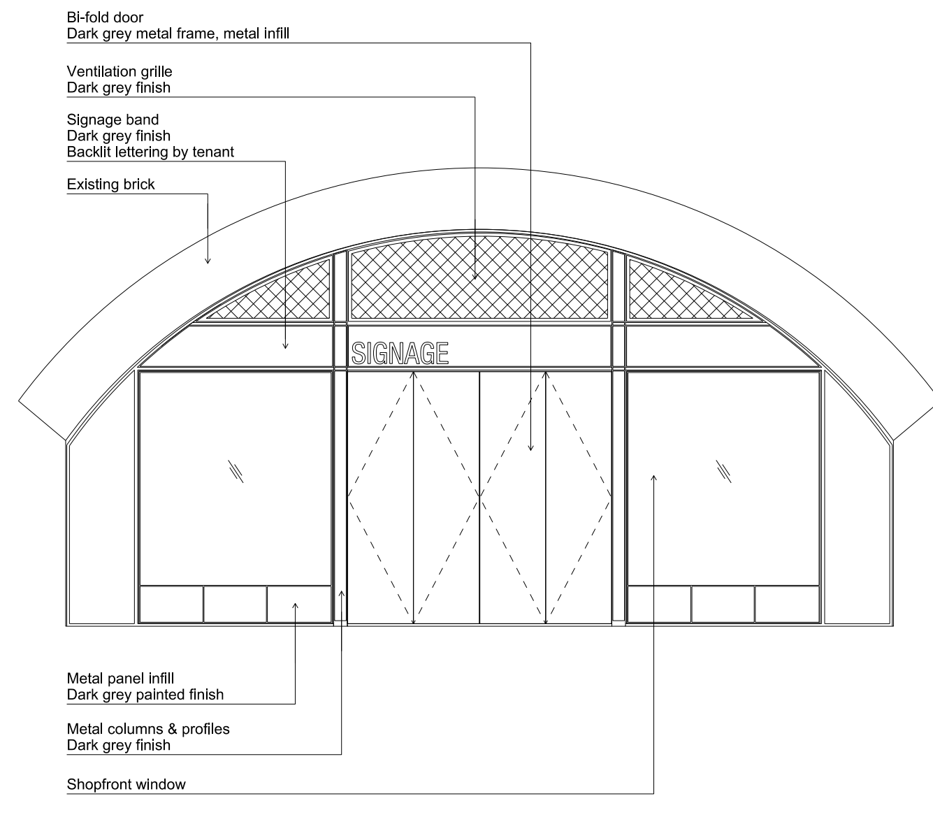
04 Retail - Single tenant SCALE 1:50
