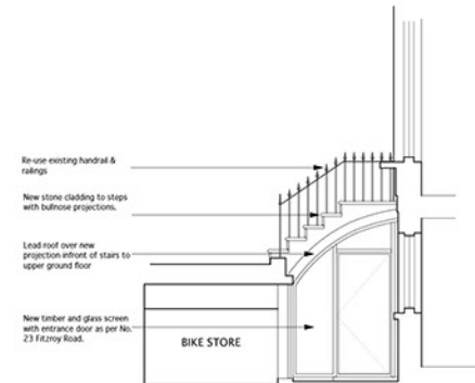
ELEVATION B
