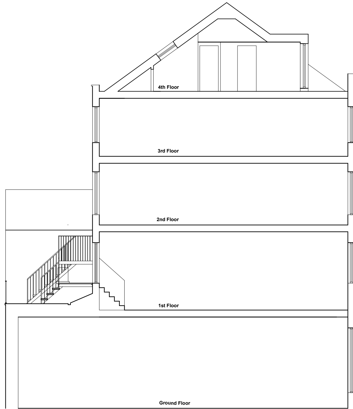
Existing Section 1:100 @ A3
