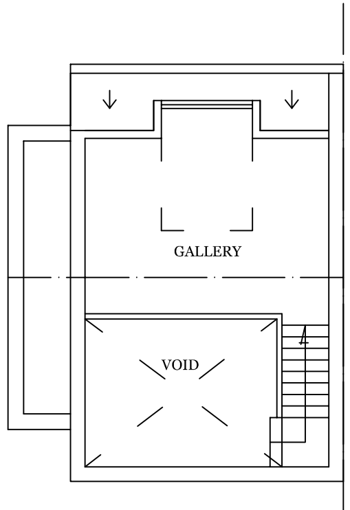
EXISTING LOFT 1:100
