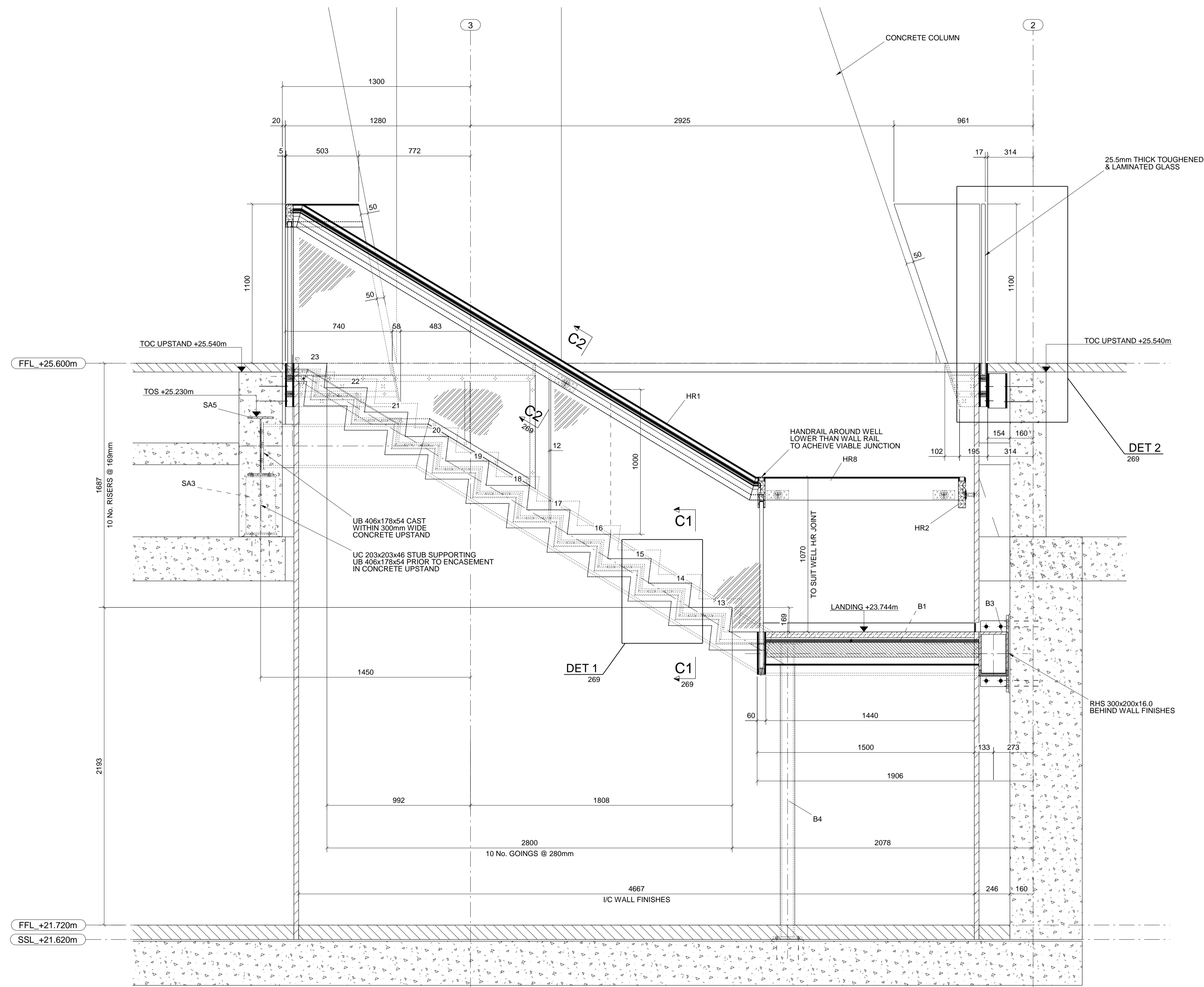
SECTION C - C E101-34-CPH-X-264
