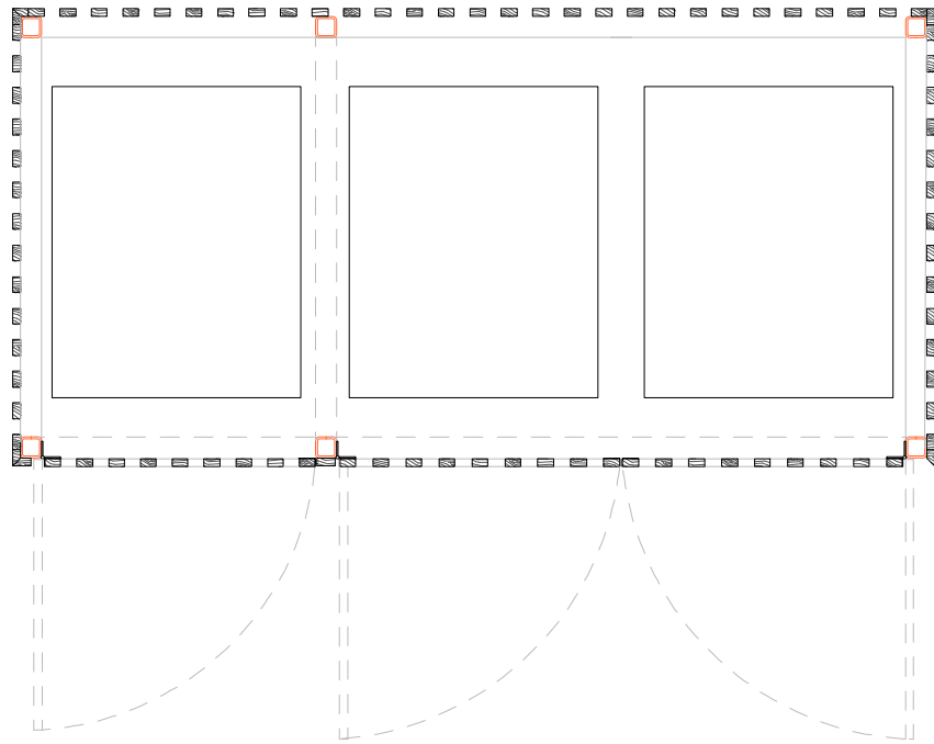
01 Plan Section 1:20
