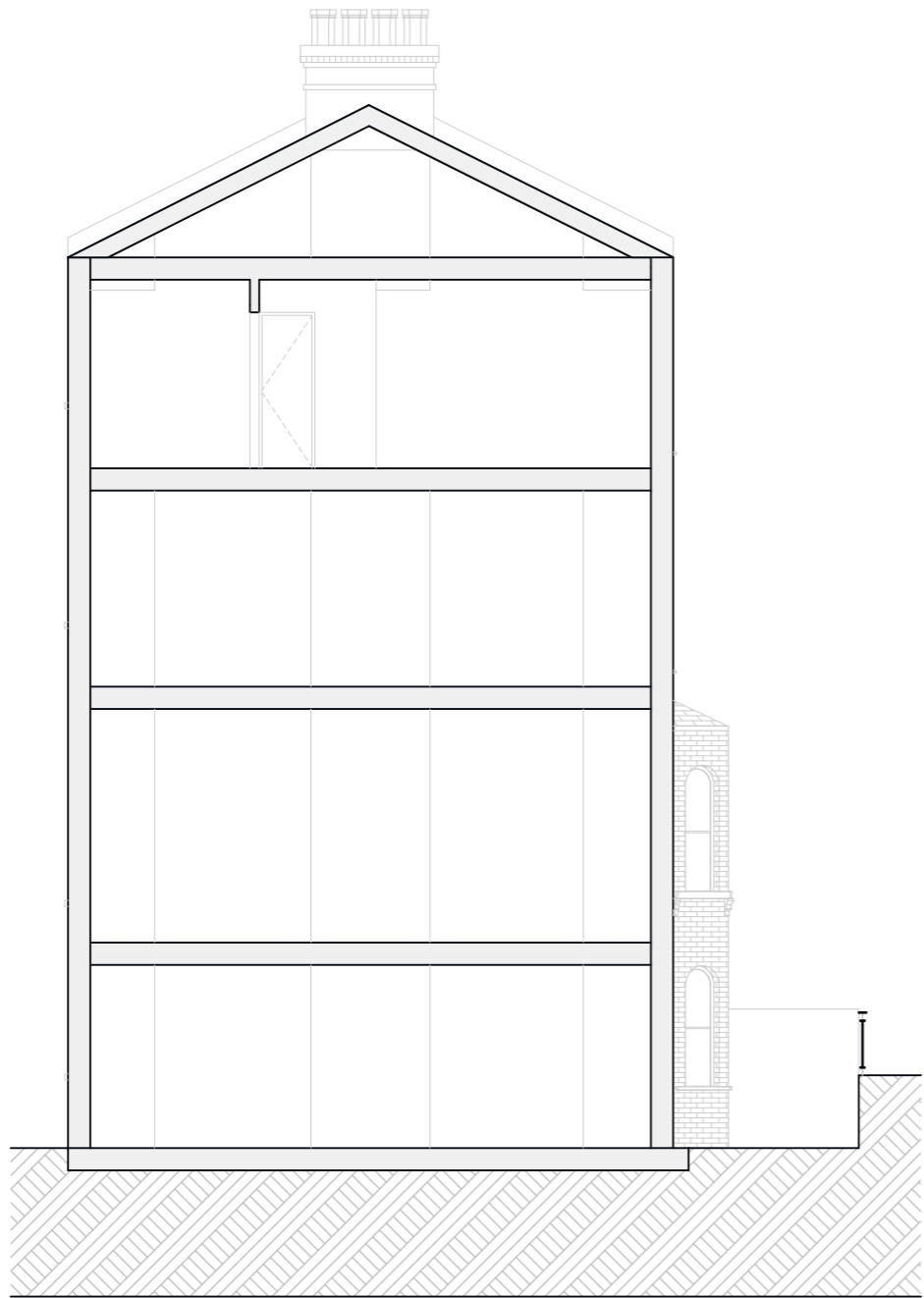
01 EXISTING LONGITUDINAL SECTION 01 1:100
