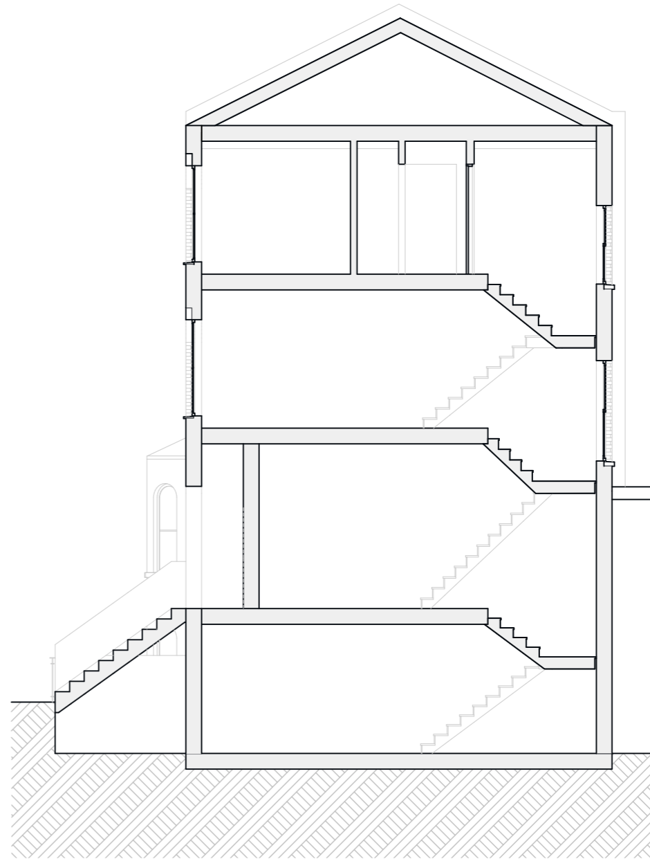
03 EXISTING LONGITUDINAL SECTION 03 1:100
