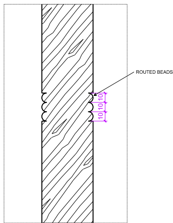
03 DOOR DETAIL
