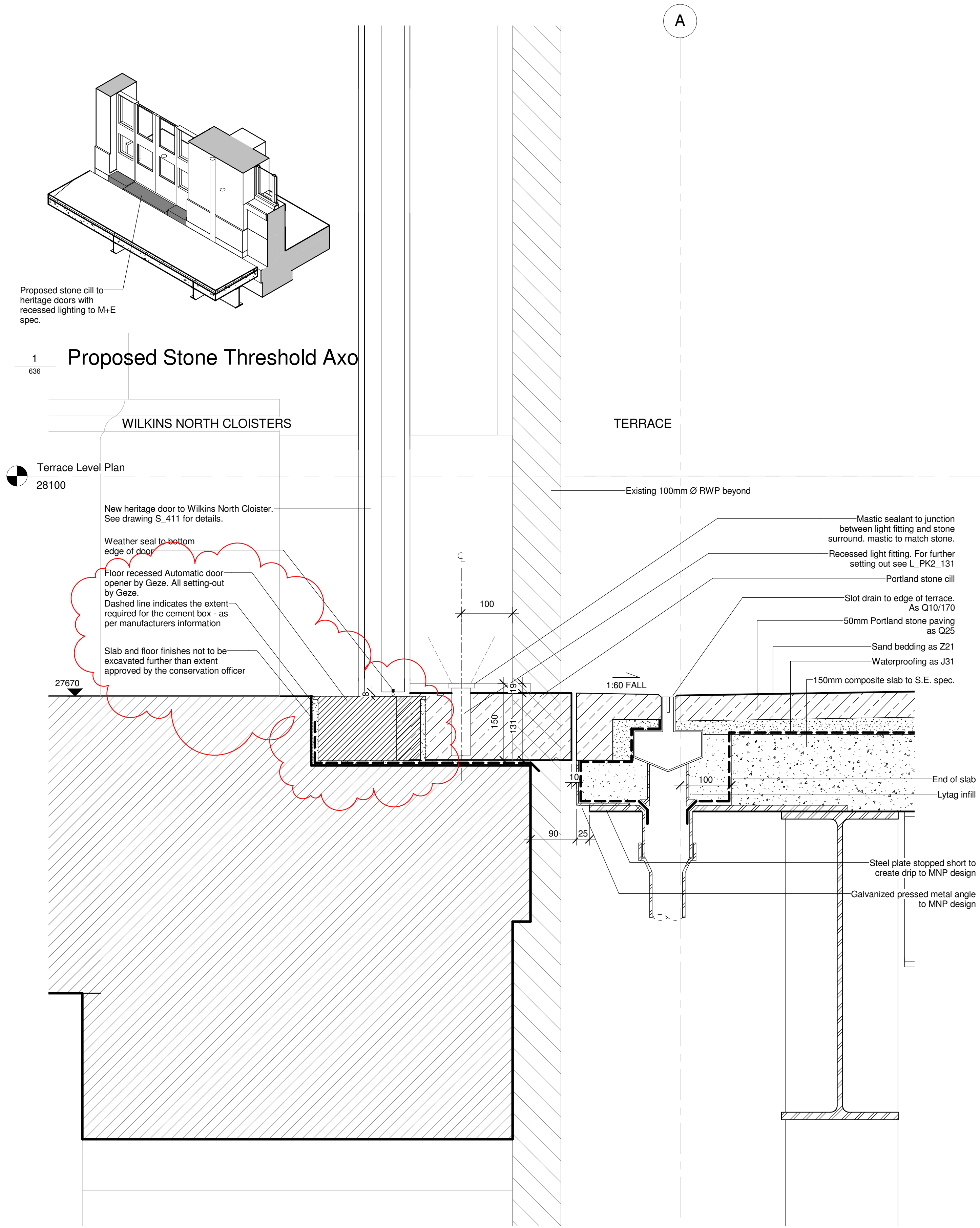
4 636 Terrace Edge Detail - Door DE30 1 : 5
