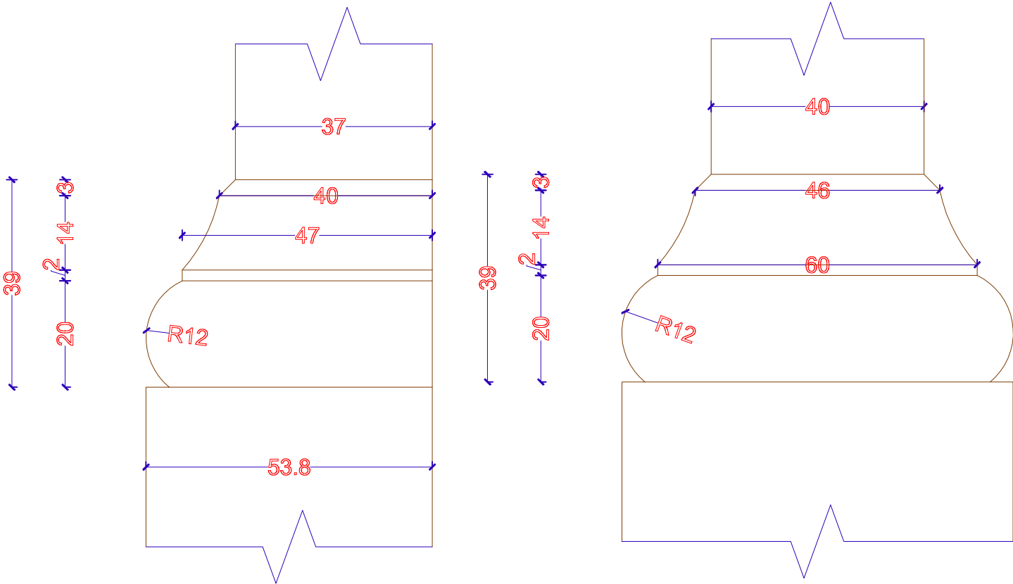
DE/29,30,31 COLUMN DETAIL LOWER SIDE sc 1:1
