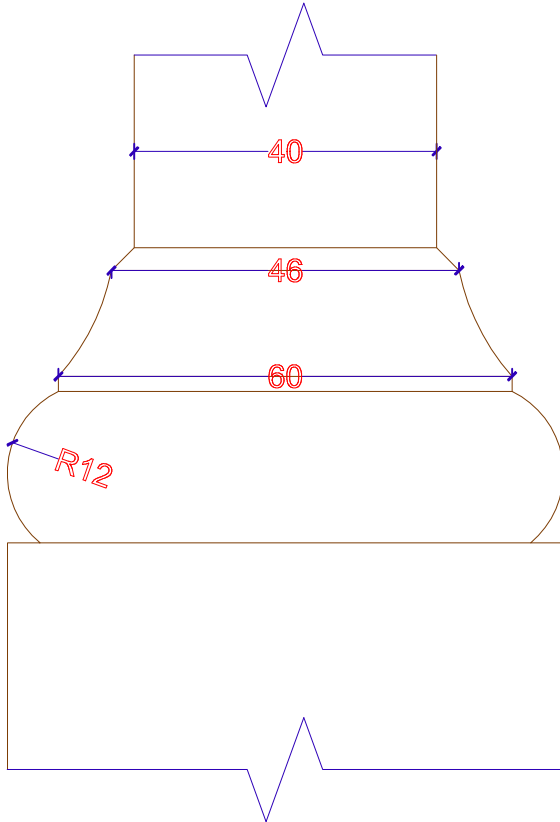
DE/29,30,31 COLUMN DETAIL LOWER SIDE SC 1:1
