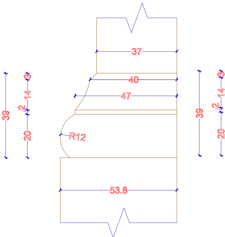
DE/29,30,31 COLUMN DETAIL LOWER SIDE SC 1:1
