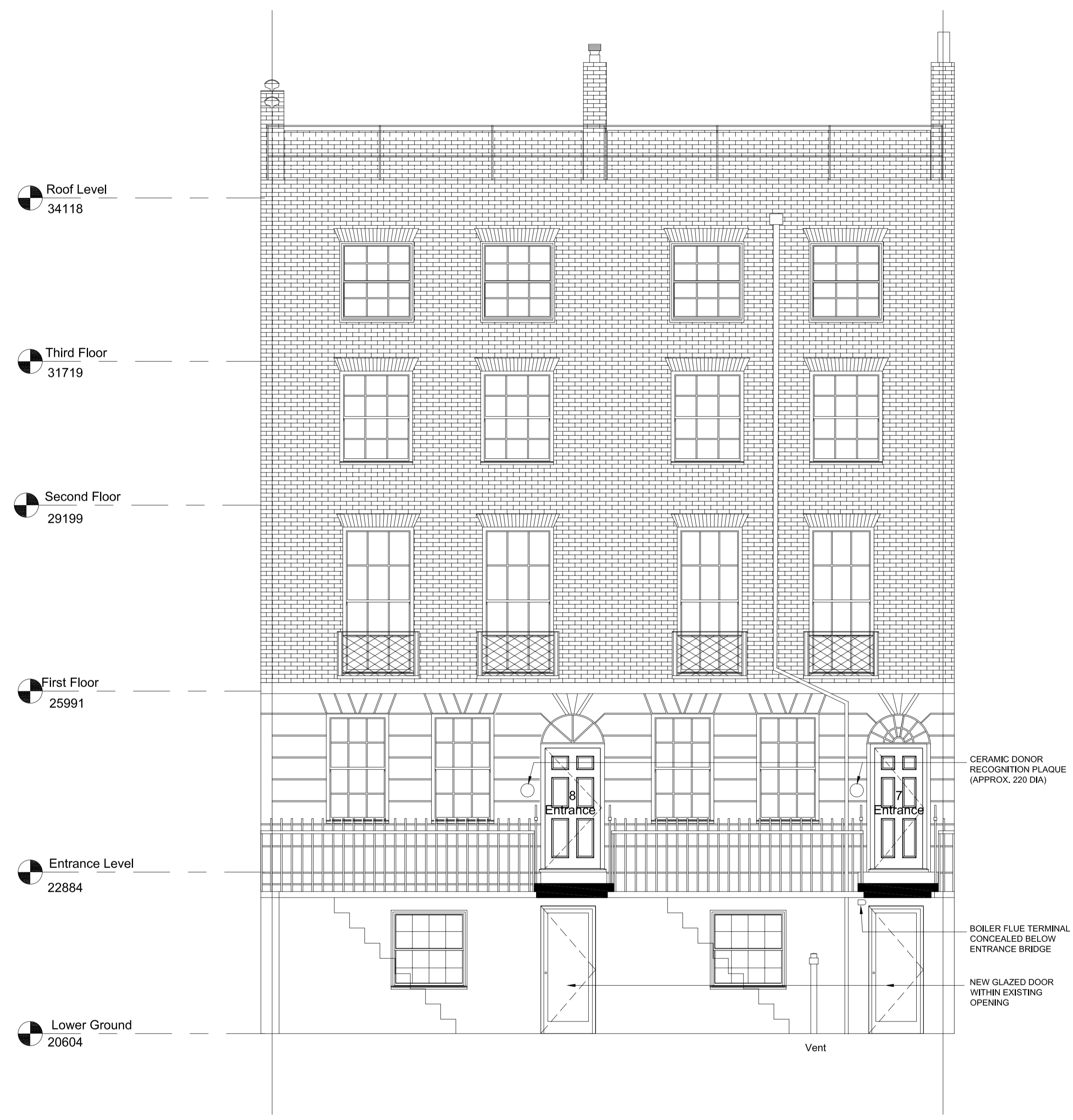
ELEVATION A
