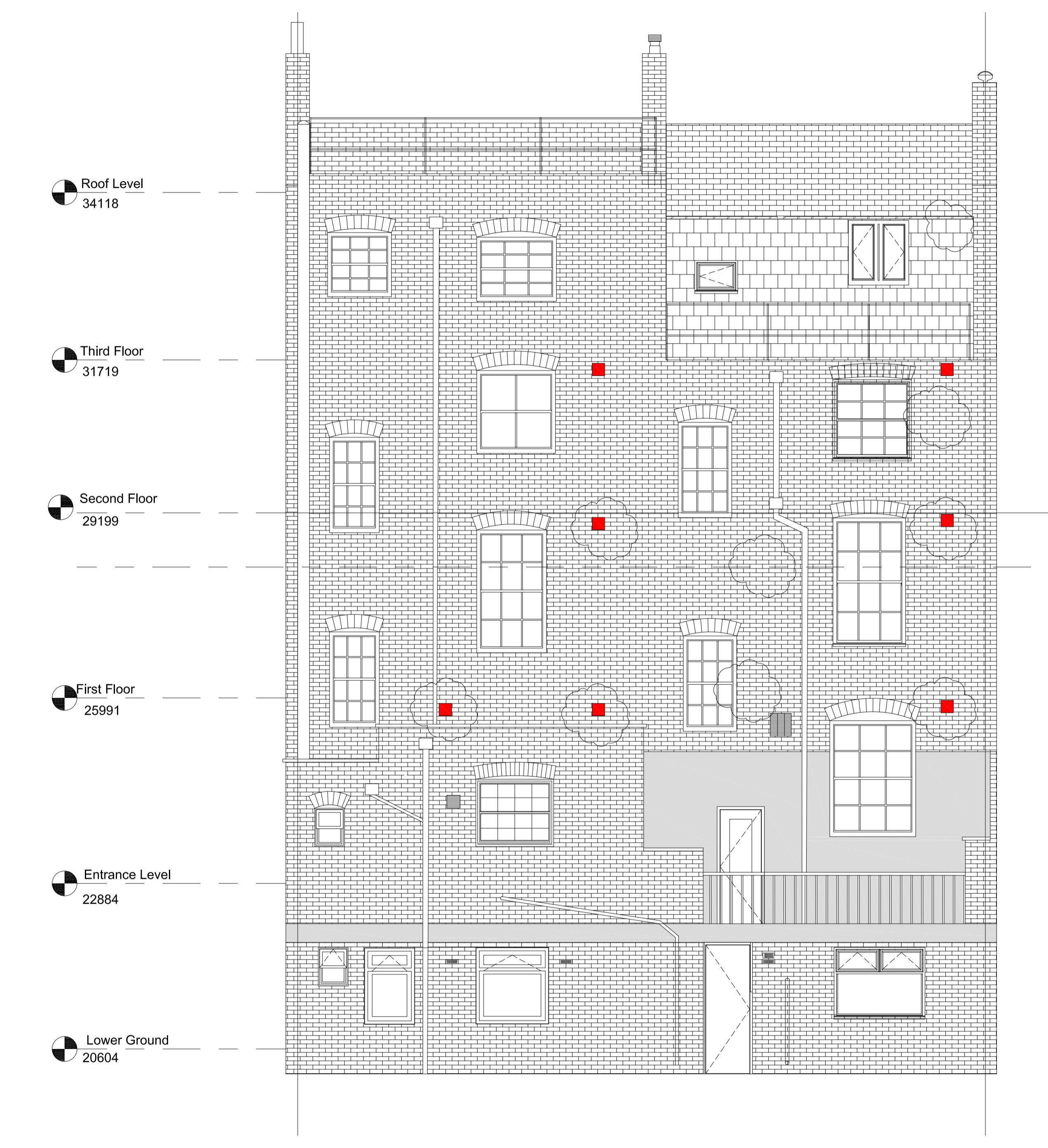
ELEVATION B
