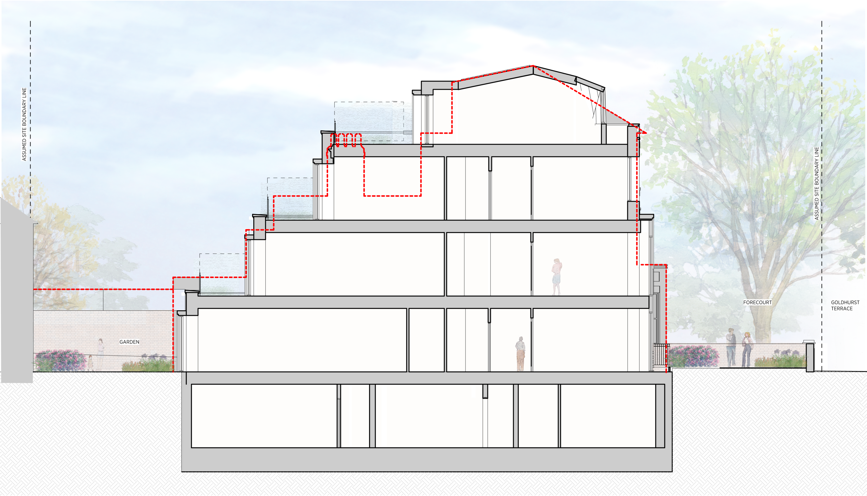
1 Section DD 1:50
