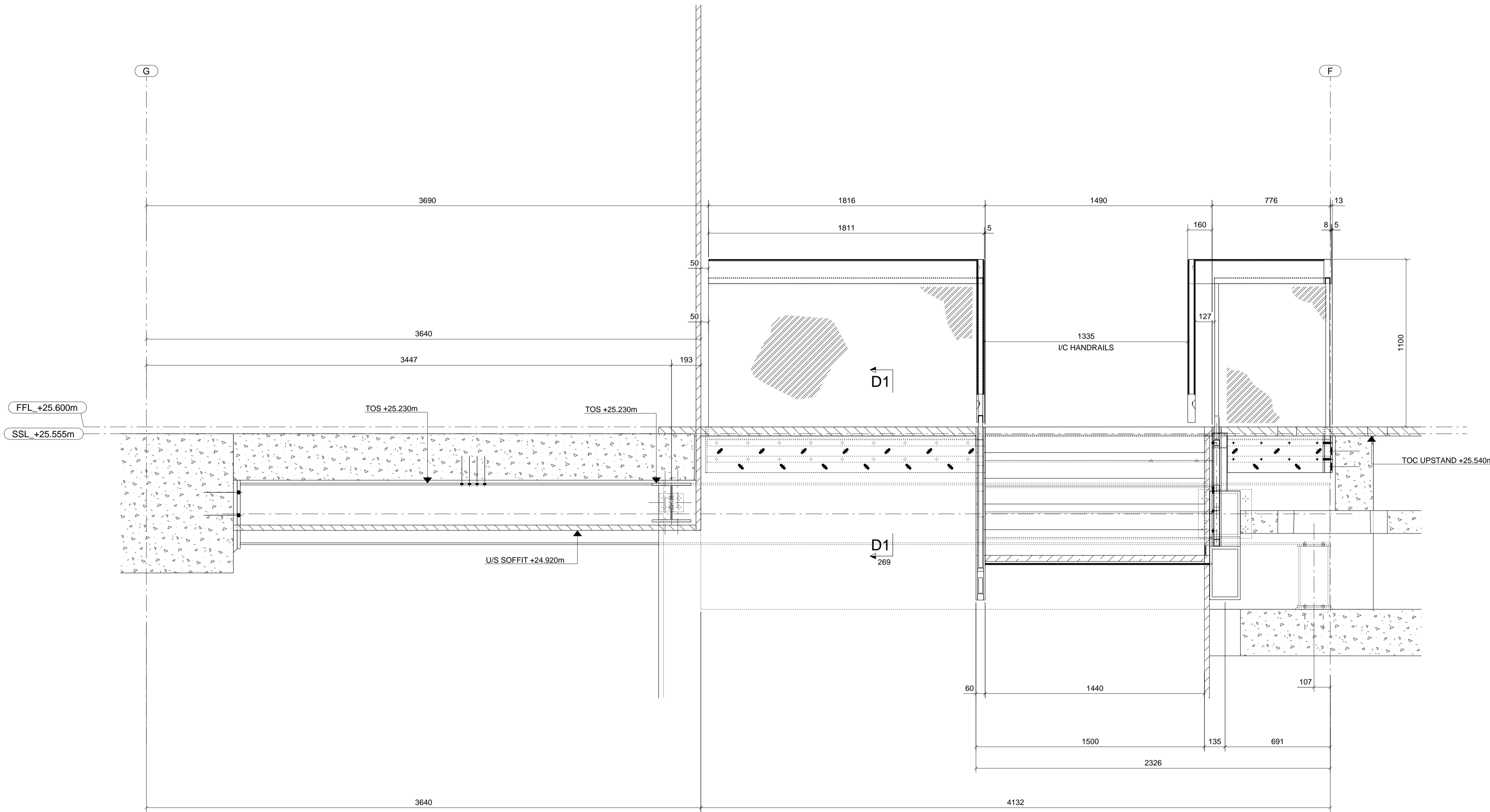
SECTION D - D E101-34-CPH-X-264
