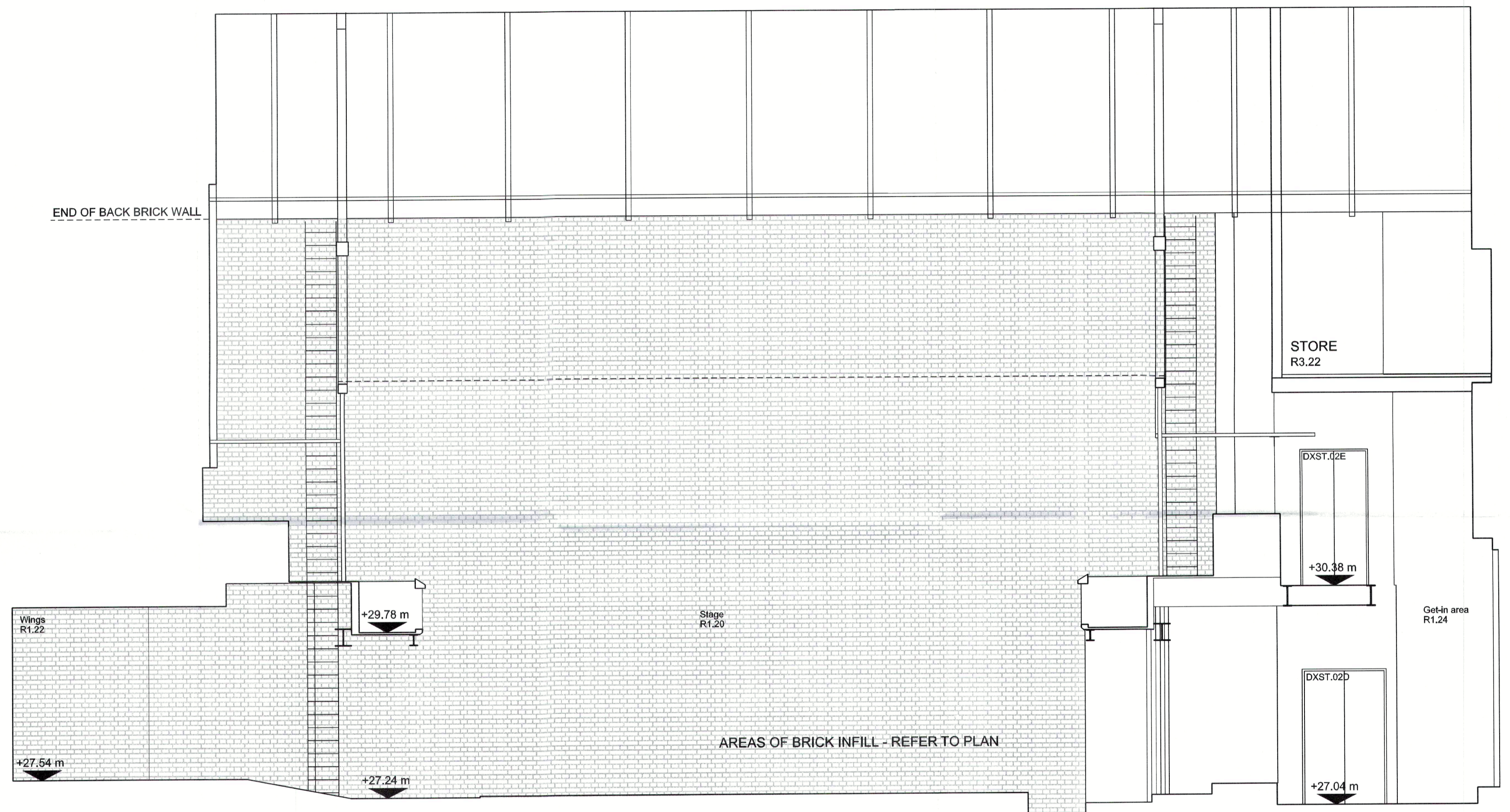
ELEVATION E1.05
