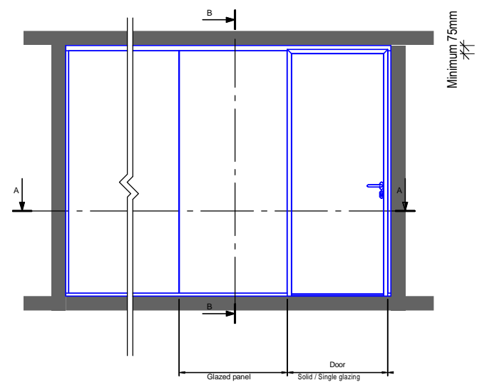
① Elevation 1 : 50
